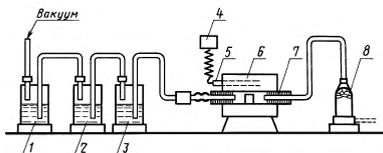
1—3 — склянки Дроксиля поглотительные; 4 — терморегулятор; 5 — термопара; 6 — печь трубчатая, электрическая, типа 1 СУОД 0,25.2,5/14К; 7 — лодочки фарфоровые; 8 — склянка Тищенко СПТ, в нижней части — безводный хлористый кальций, в верхней — кусочки гидроокиси натрия
