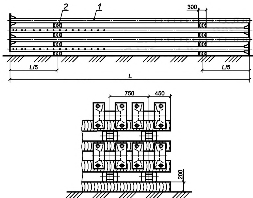
Рисунок Д.2 — Схема хранения стоек металлических
