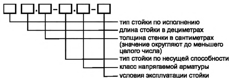
Рисунок Б.1 — Пример условного обозначения стоек железобетонных
