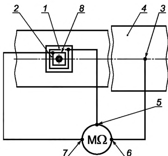
1 — изолирующий элемент; 2 — стальная шайба; 3 — выпуск провода диагностики; 4 — стойка; 5 — клемма «Экран» мегаомметра; 6 — клемма «Земля» мегаомметра; 7 — клемма «Линия» мегаомметра; 8 — экран из медной проволоки диаметром 3 мм
