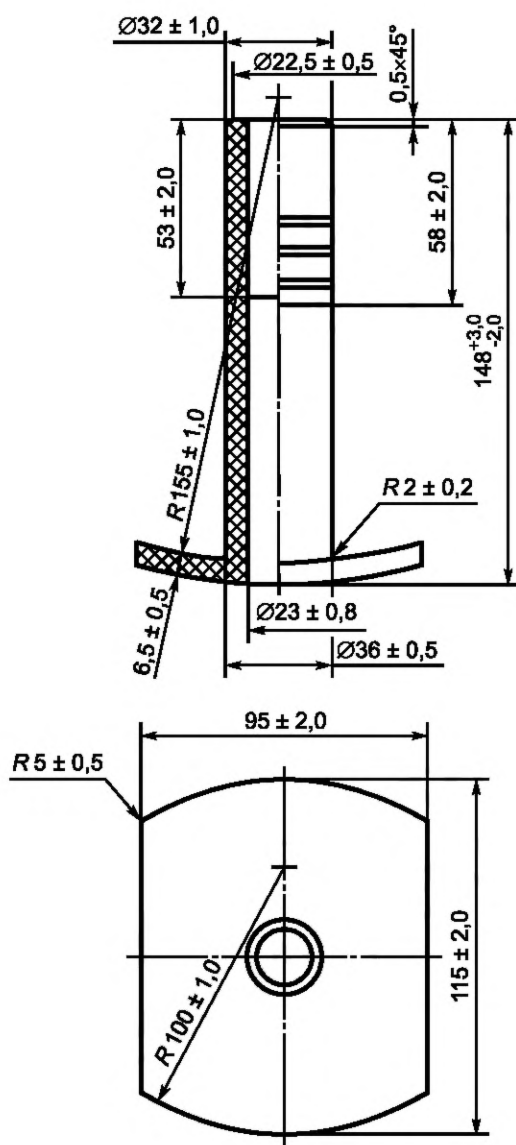
Рисунок А.6 — Втулка изолирующая съемная В-2
