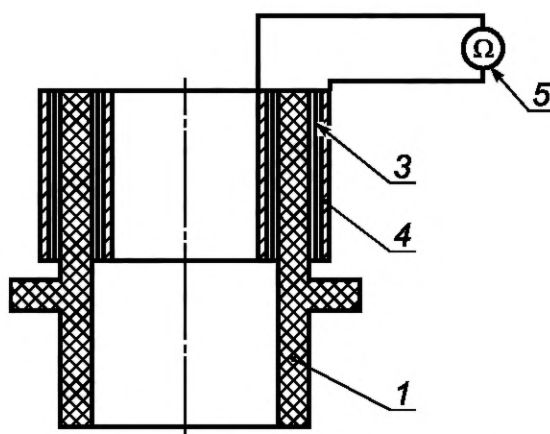
а) схема измерения объемного электрического сопротивления втулки
