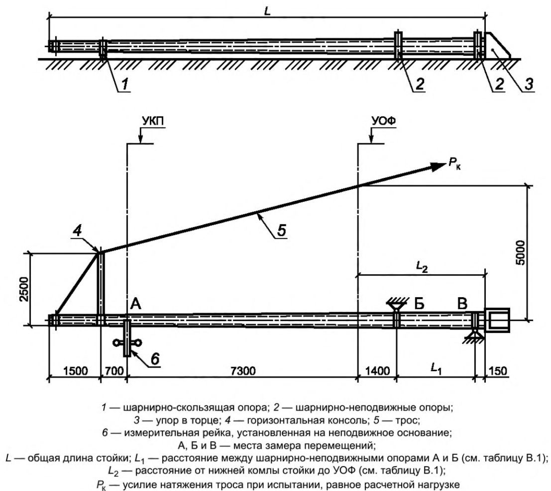
Рисунок В.1 — Схема механических испытаний стоек железобетонных 1-го типа по исполнению, закапываемых непосредственно в грунт
