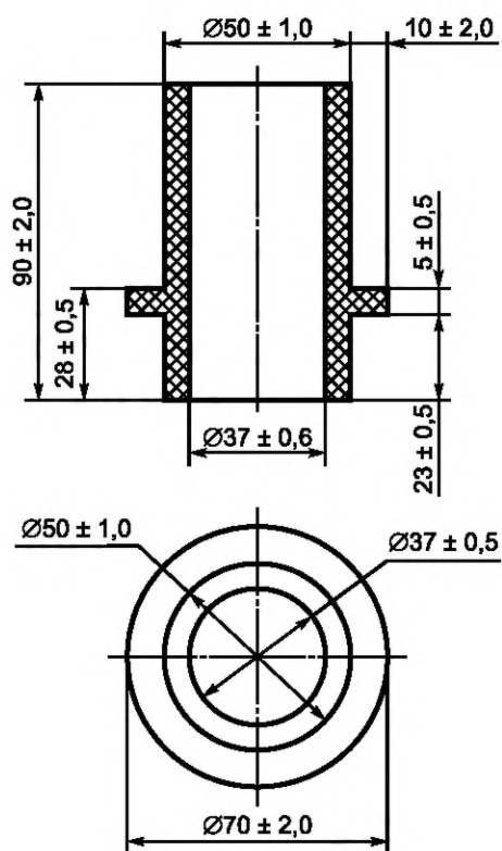
Рисунок А.5 — Втулка изолирующая несъемная В-1
