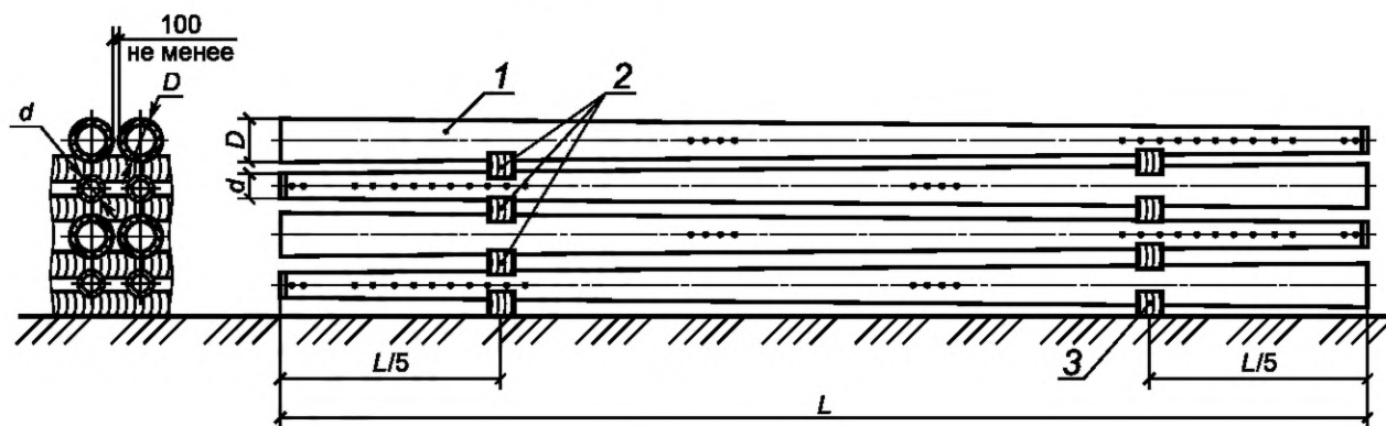
а) схема штабеля
