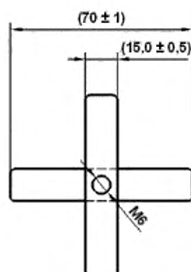
Рисунок 4 – Лопасты мешалки
