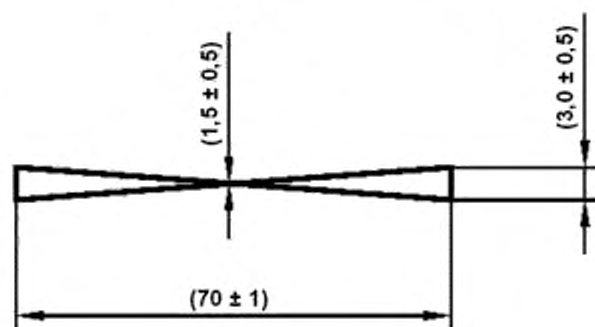
Рисунок 5 – Размеры лопастей мешалки
