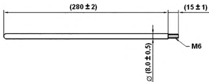
Рисунок 3 – Типовой шток мешалки
