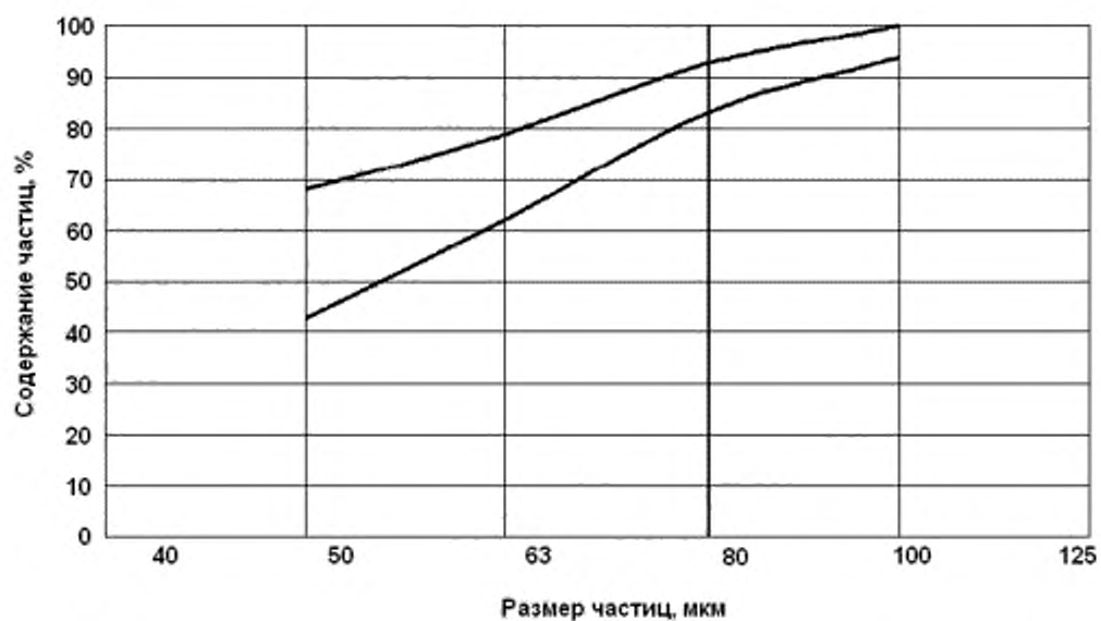
Рисунок А.1 – Типичный гранулометрический состав наполнителя Сикесол
