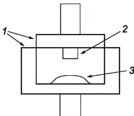
1 — каркас для сжатия; 2 — плунжер; 3 — испытываемый образец
