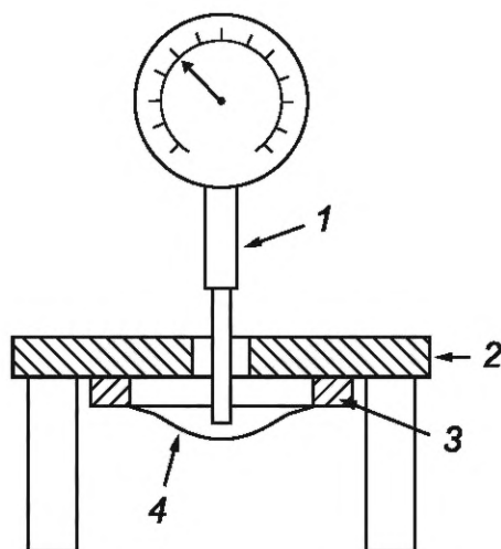
1 — толщиномер (4.6.1.2); 2 — плоская плита (4.6.1.1); 3 — зажимное кольцо; 4 — испытываемый образец
