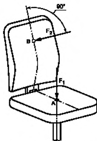
A — точка нагружения; B — точка нагружения спинки; F 1 — вертикальная нагрузка; F 2 — горизонтальная нагрузка
