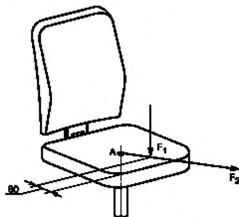
Рисунок 9 — Опрокидывание вперед
