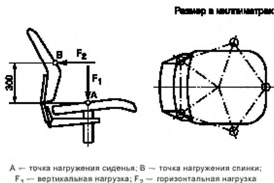
Рисунок 12 — Испытание спинки на опрокидывание назад для стульев без наклона спинки
