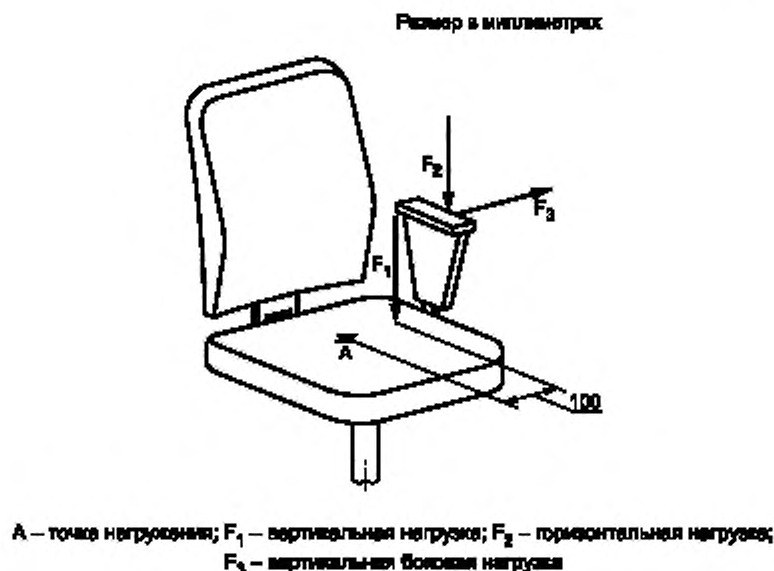
Рисунок 11 — Боковой наклон стула с подлокотниками
