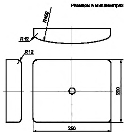
Рисунок 3 — Подушка для нагружения спинки
