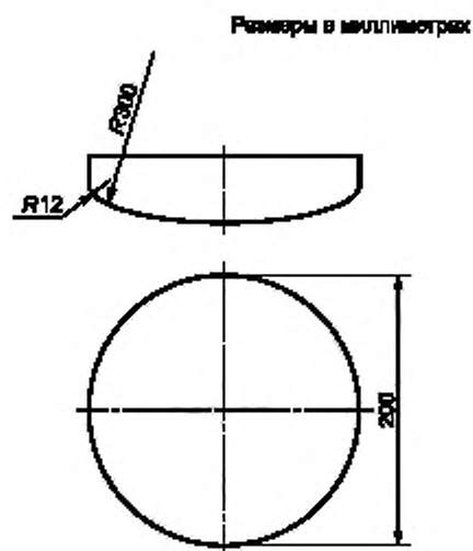
Рисунок 2 — Малая подушка для нагружения
