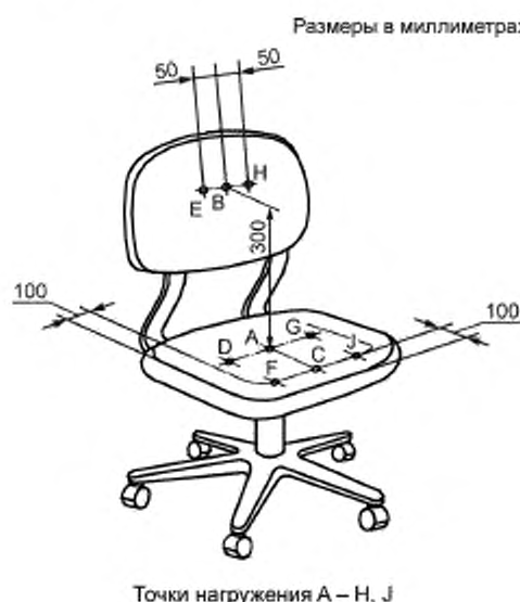
Рисунок 7 — Точки нагружения
