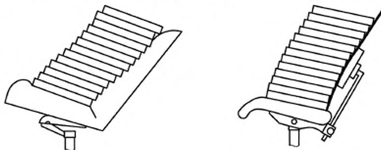
Рисунок 13 — Испытание спинки опрокидывание назад для стульев с наклоном спинки
