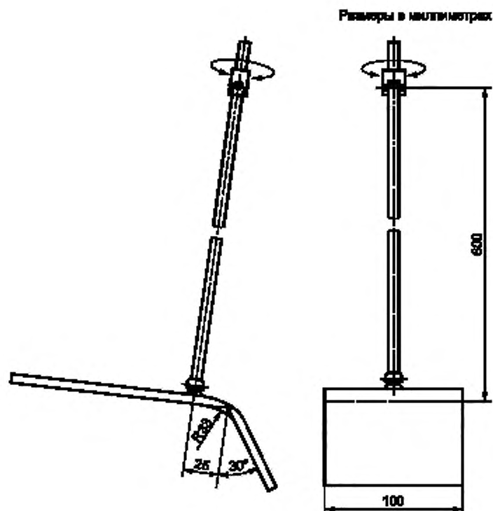
Рисунок 5 — Образец подушки нагружения подлокотника
