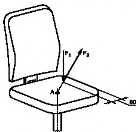
А — точка нагружения; F_1 — вертикальная нагрузка; F_2 — горизонтальная нагрузка
