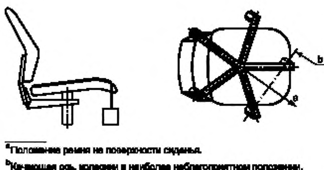
Рисунок 8 — Опрокидывание переднего края
