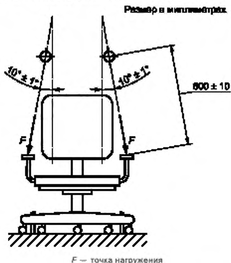
Рисунок 4 — Принцип работы устройства для испытания на прочность подлокотников
