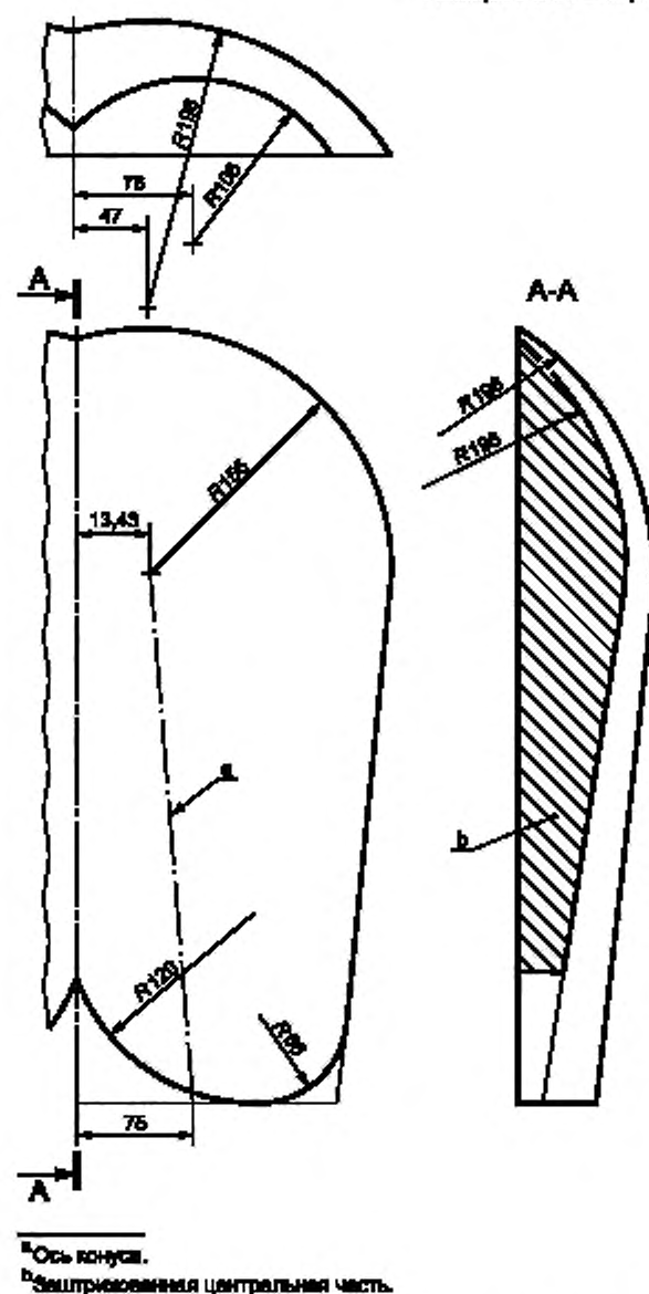
Рисунок В.1 — Линейные размеры подушки нагружения — Конструкция из древесины твердых пород
