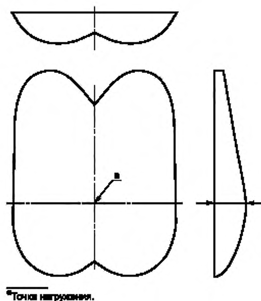
Рисунок 1 — Подушка для нагружения
