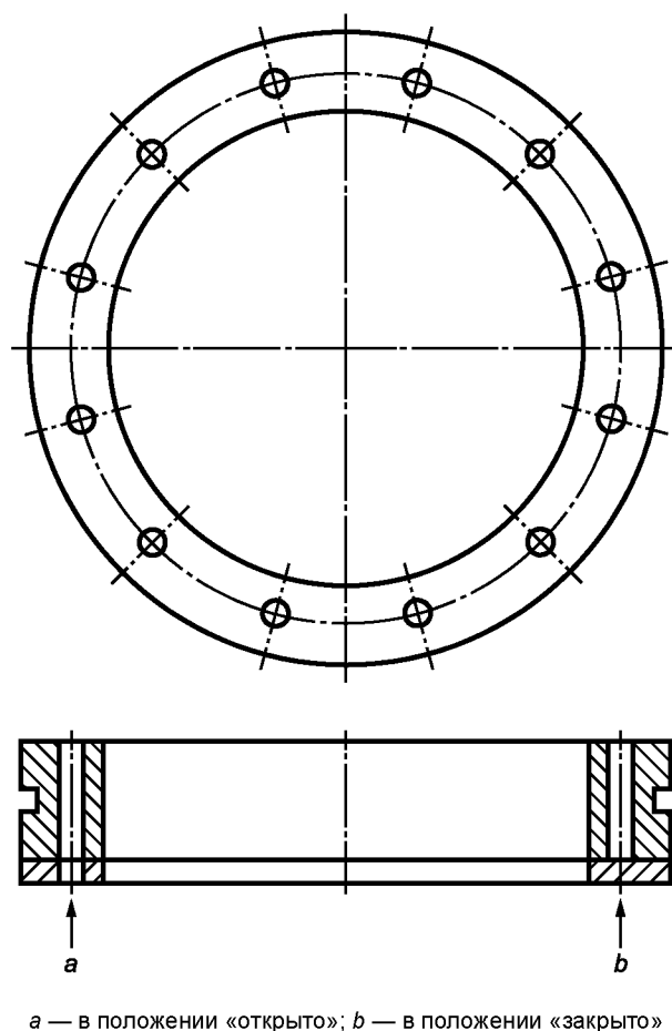
Рисунок А.1 — Регулируемый обжимной хомут (нижняя часть обжимного хомута регулирует расход воздуха через капюшон)
