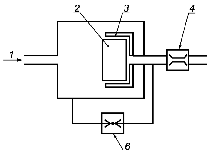
б) Держатель для испытания фильтров
