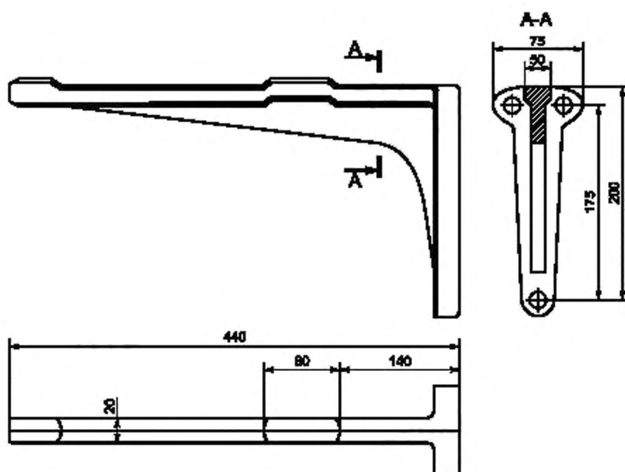
Рисунок 3 — Кронштейн чугунный для мойки, большой
