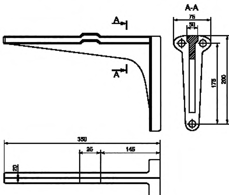
Рисунок 4 — Кронштейн чугунный для мойки, малый
