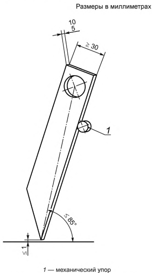
Рисунок 8 — Противоосколочный палец
