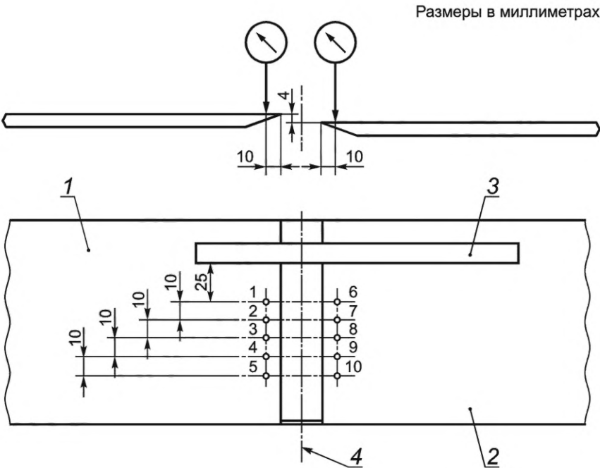
1 — приемный стол; 2 — подающий стол; 3 — направляющее ограждение; 4 — ось строгальной ножевой головки Рисунок G.3 — Точки измерения шероховатости столов
