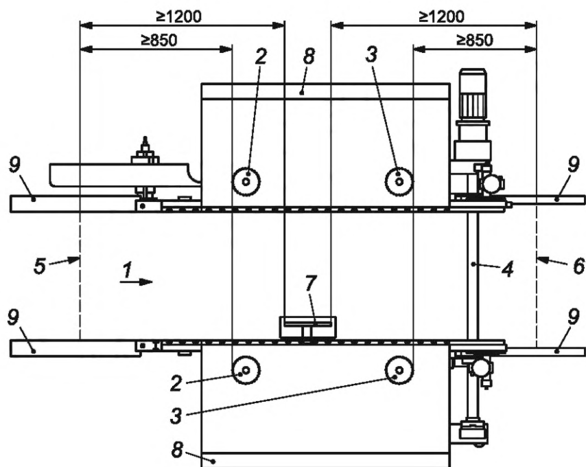
1 — направление подачи; 2 — первые инструменты; 3 — последние инструменты; 4 — приводной вал; 5 — AOPD на входной стороне станка; 6 — AOPD на выходной стороне станка; 7 — узел фрезерования канавок, установленный вне корпуса; 8 — корпус станка; 9 — опора заготовки
