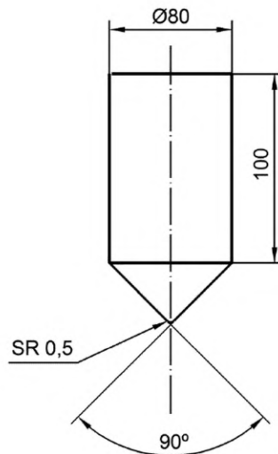
Рисунок 1 — Испытательный конус
