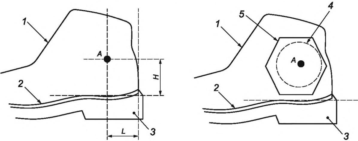
1 — верх; 2 — вкладки/основная стельки; 3 — подошва; 4 — минимальный диаметр области защиты лодыжки; 5 — защитная область лодыжки; L — измеренное расстояние от свода до края подошвы; H — измеренная высота от свода до лодыжки
