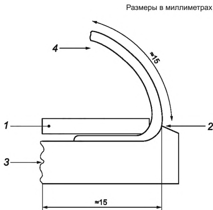
Рисунок 3 — Поперечное сечение испытуемой пробы
