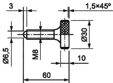
Рисунок 10 — Пример регулировочного винта
