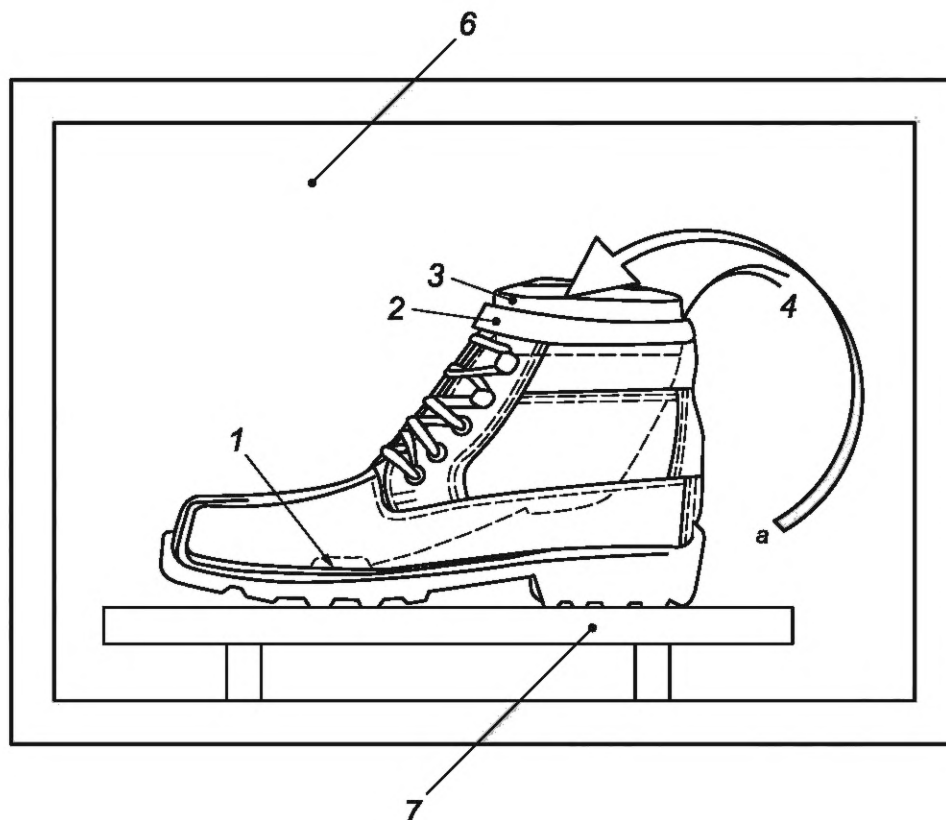
1 — точка измерения температуры; 2 — лента; 3 — заглушка; 4 — провода к термопаре; 6 — холодильная камера; 7 — медная пластина (см. 5.16.1.5); а — заполняющие стальные шарики (здесь не показаны)
