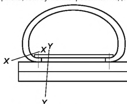
Тип f — Машинная прошивка подошвы или ранта с подошвой, где подошва прикреплена к подложке
