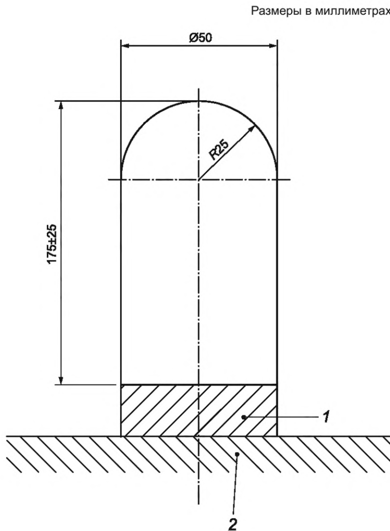
Рисунок 28 — Наковальня и основание
