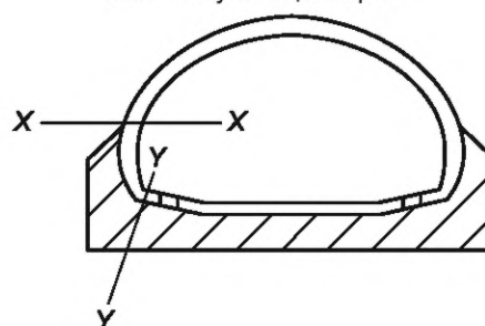
Тип b — Стандартная затяжка, подошва без выступающего края
