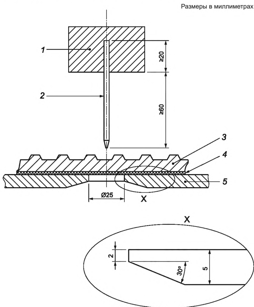
1 — система зажима гвоздя; 2 — гвоздь; 3 — подошвенный узел из испытуемой пробы; 4 — антипрокольная прокладка; 5 — пластина
