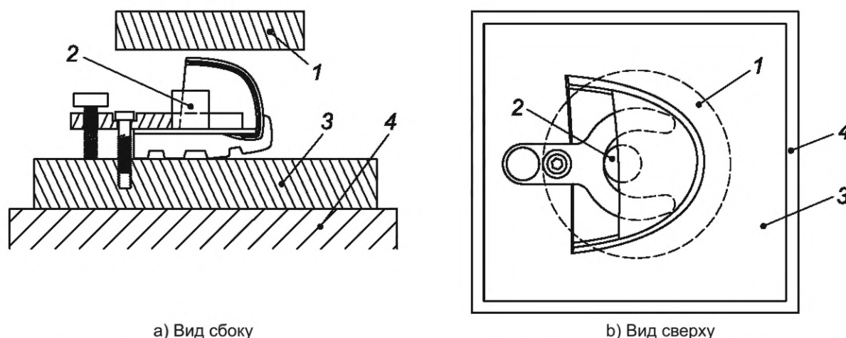
Рисунок 14 — Принцип работы установки для определения сопротивления сжатию (пример конструкции)
