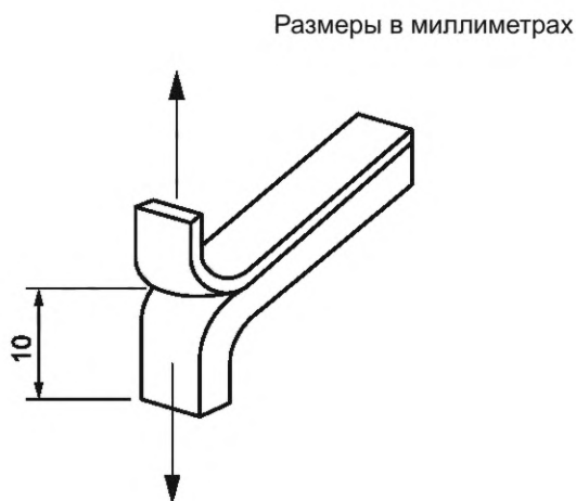
Рисунок 4 — Подготовленная испытуемая проба
