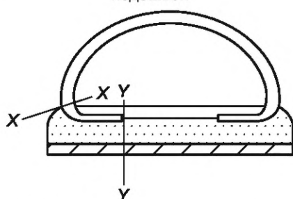
Тип g — Многослойная подошва, например приливка на подошву, литевой элемент или составной элемент
