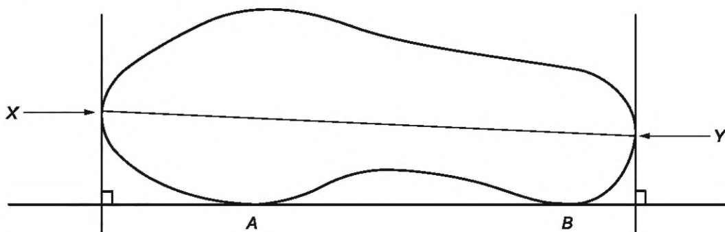
Рисунок 12 — Испытательная ось для обуви
