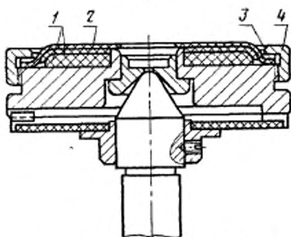
1—эластичное основание; 2—токопроводящая резина; 3—металлическое кольцо; 4—обойма.
