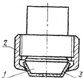
1—грибок; 2—обойма; 3—ткань.
