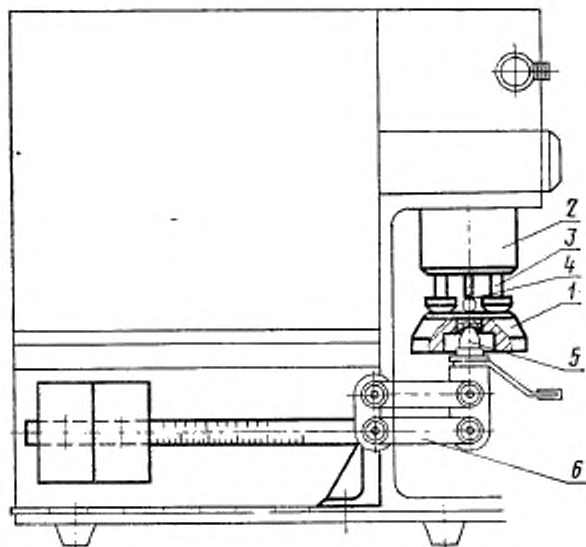
1—пальцы; 2—испираторная головка; 3—бегунок; 4—устройство для натяжения используемой или образцовой ткани; 5—опора пальцев; 6—рычажно-грузовая система для создания нормального давления.
