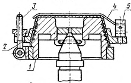
1—пила; 2—кольцо; 3—откидной винт; 4—контактная проволока; 5—пружина.
