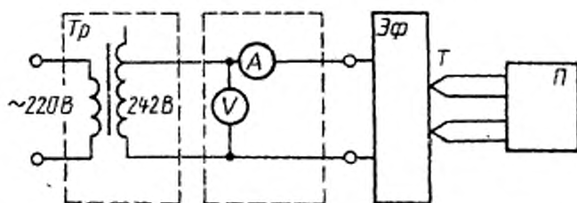
Тр — регулятор напряжения РНО; ЭФ — испытуемый фен; П — автоматический потенциометр КП-4; Т — термозлектрический преобразователь ТХА
