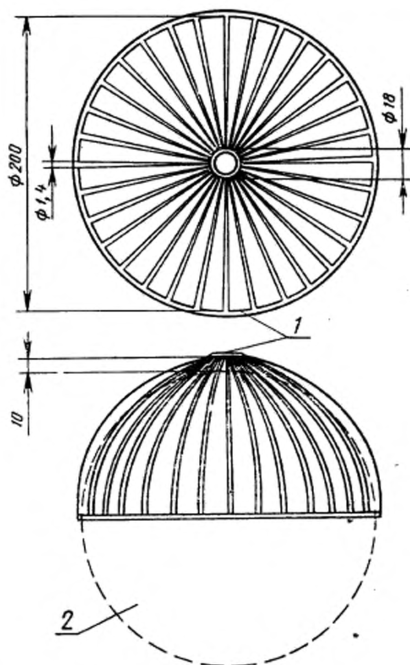
Защитное устройство из металлической проволоки
