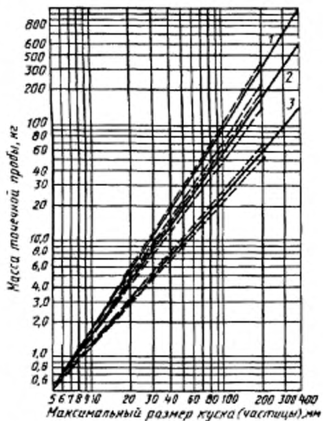
Рисунок А.1 — Масса точечной пробы в зависимости от номинального верхнего размера частиц ферросплавов
