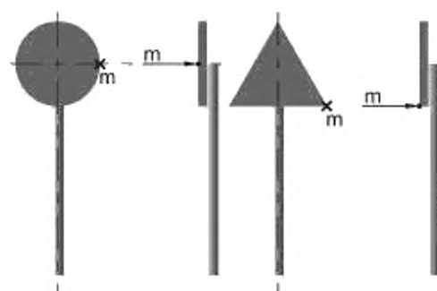
Рисунок A.4 — Схема приложения горизонтальной точечной нагрузки
