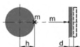
Рисунок A.5 — Схема измерения максимального временного отклонения конструкции дорожного знака
