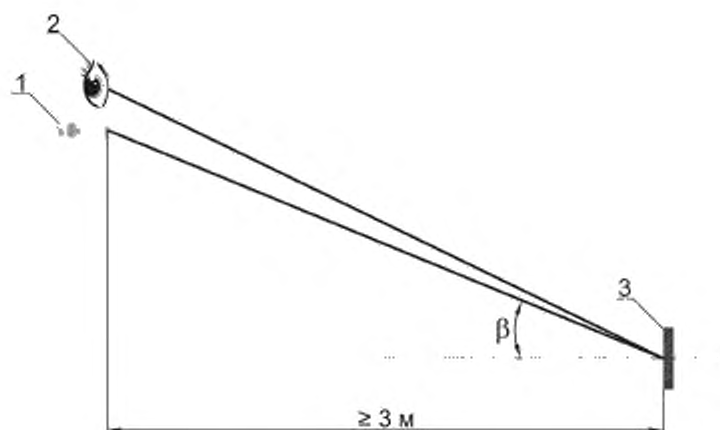
1 — стандартный источник света типа А; 2 — фотоприемник; 3 — образец световозвращающего материала; \beta — угол освещения
