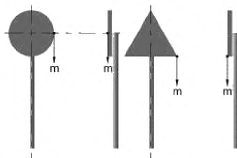
Рисунок A.3 — Схема приложения вертикальной точечной нагрузки
