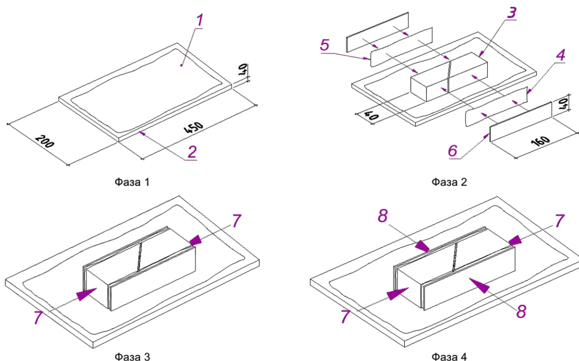
Рисунок В.1 — Схема склеивания в кондукторе контрольных образцов-призм с наклонным клеевым швом
