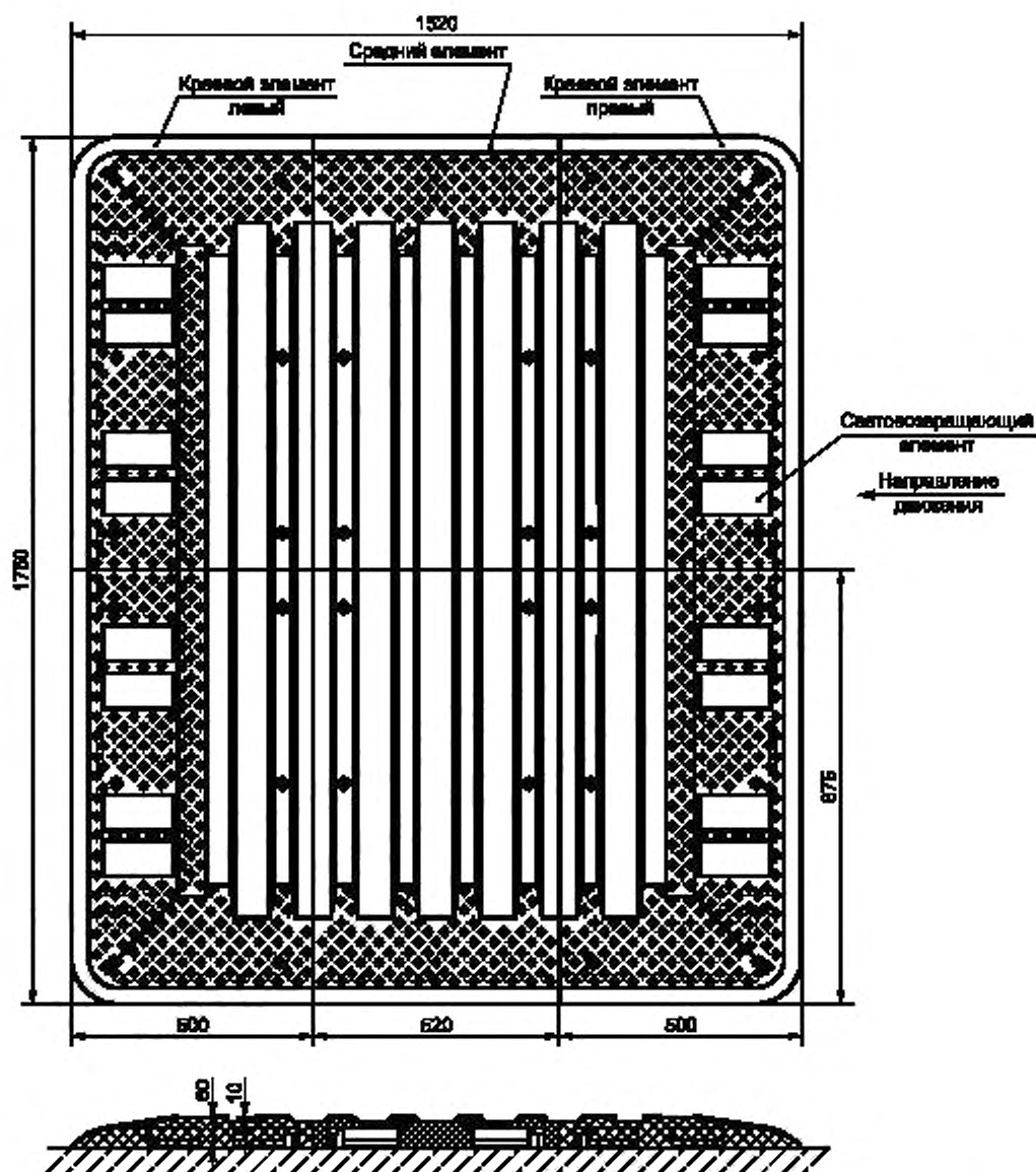
Рисунок Б.2 — Пример конструкции ИНС, устраиваемых на полосе движения безрельсового общественного транспорта
