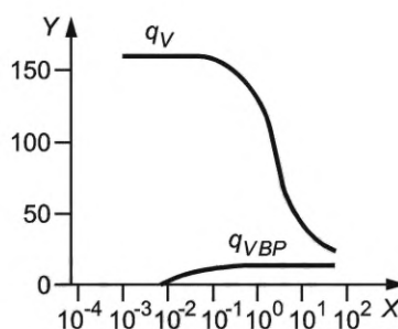
X — выпускное давление, Па; Y — быстрота действия л/с; q_V — быстрота действия испытуемого насоса; q_{VBP} — быстрота действия форвакуумного насоса
