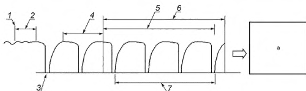
Рисунок Р.6 — Испытание теплопроводности с двумя полными циклами в течение периода сбора данных
