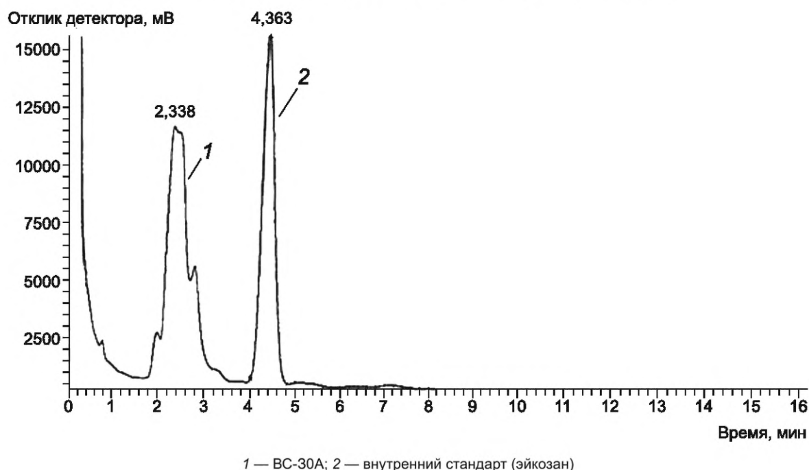
Рисунок 1 — Хроматограмма определения антиоксиданта ВС-30А
