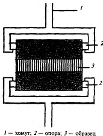
Рисунок В.1 — Схема закрепления образца в универсальном зажимном устройстве
