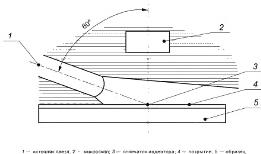
Рисунок 13 — Расположение источника света и микроскопа при проведении испытаний
