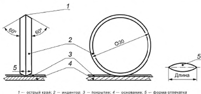
Рисунок 12 — Схема проведения испытания
