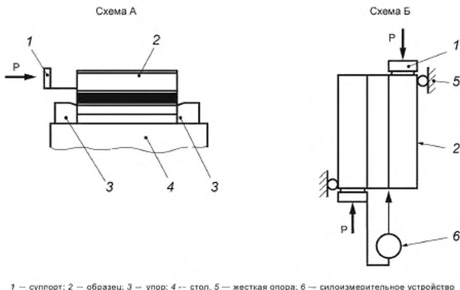
Рисунок А.2 — Схема приложения сдвигающей нагрузки
