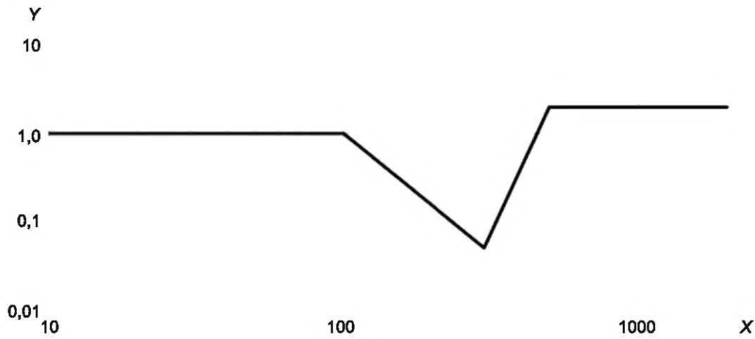
Y — ASD [(м/с²)²/Гц]; X — частота, Гц Рисунок 1 — ASD случайной вибрации
