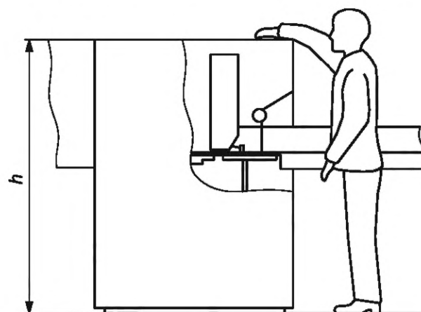
Рисунок 5 — Высота переднего ограждения
