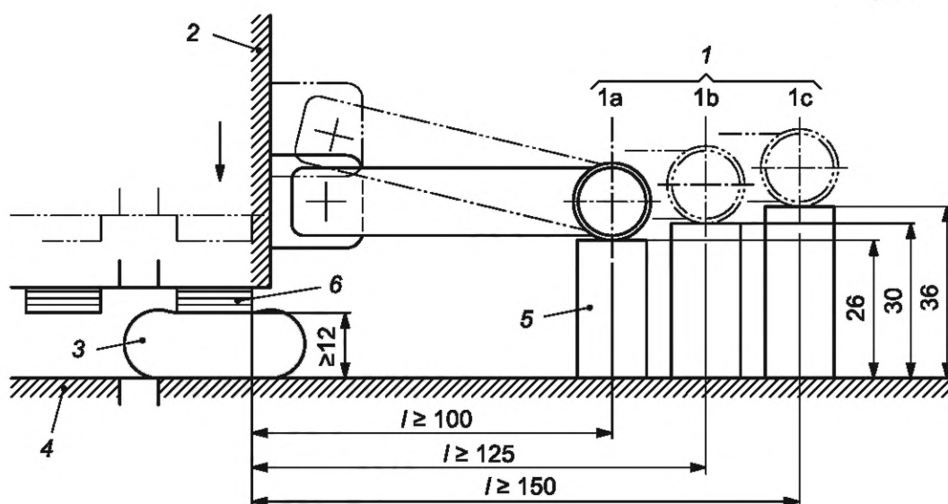
1 — возможные положения датчика полосы отключения: 1a, 1b, 1c; 2 — прижимная балка; 3 — моделирующий пластилиновый блок; l — горизонтальное расстояние датчика полосы отключения до позиции 6; 4 — опора заготовки; 5 — жесткий дистанционный блок; 6 — нижняя жесткая часть прижимной балки
