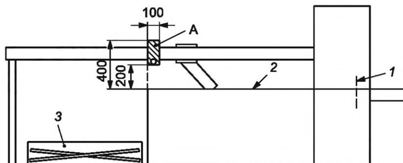
1 — линия резания; 2 — стол станка; 3 — подъемный стол; A — область для AOPD 2
