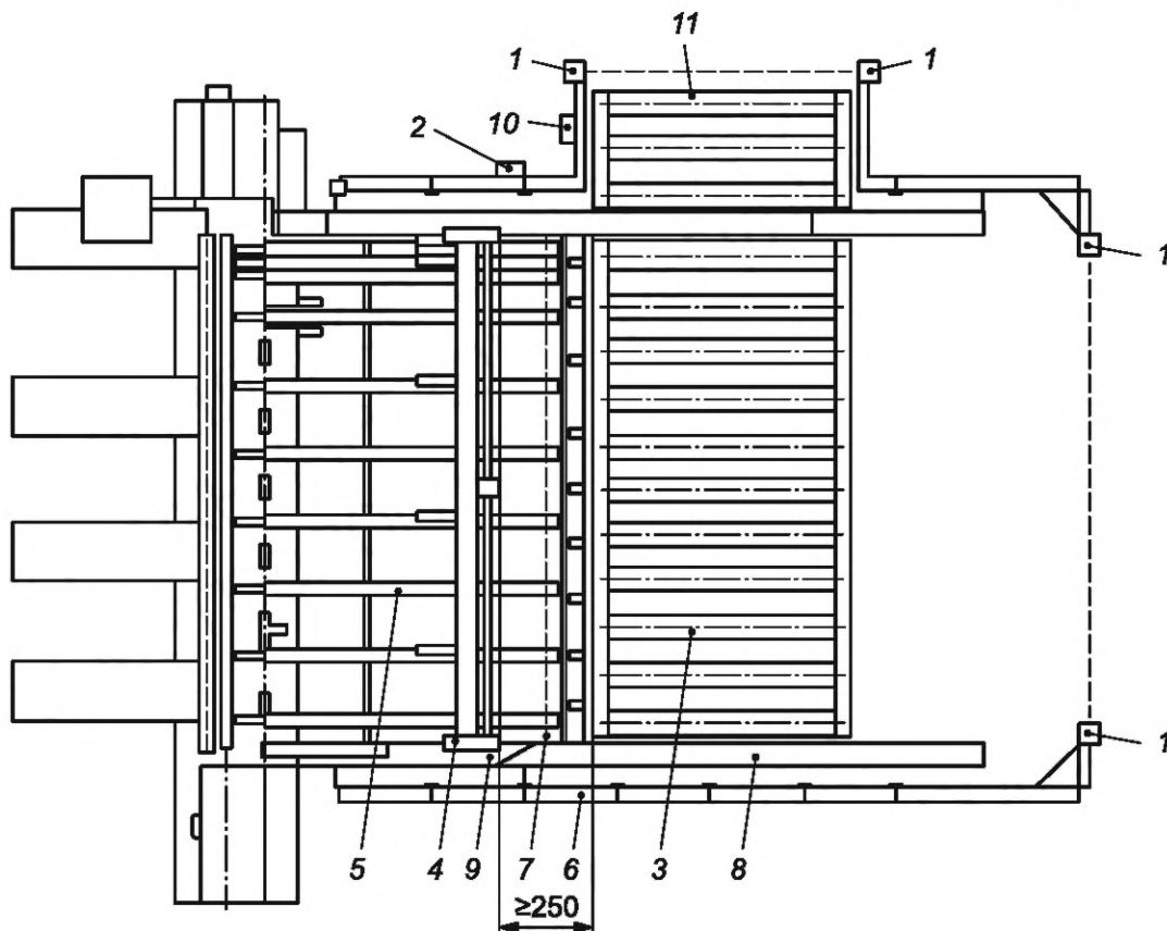
1 — AOPD 1; 2 — орган управления сбросом для подъемной платформы AOPD 1; 3 — подъемная платформа; 4 — толкатель панели; 5 — опора для заготовки станка; 6 — заднее ограждение; 7 — AOPD 2; 8 — предохранительный механический кулачок; 9 — предохранительный выключатель; 10 — держатель для органа управления; 11 — роликовый конвейер
