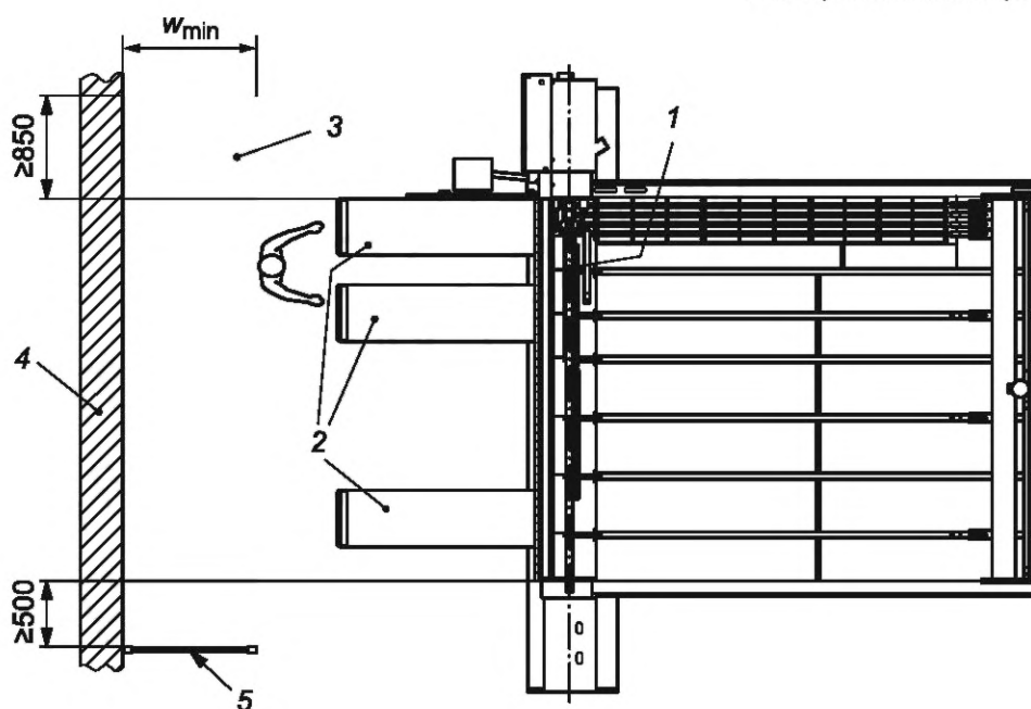
1 — передняя линия резания; 2 — удлинительные столы; 3 — ESPE или чувствительные к давлению маты; 4 — стена; 5 — ограждение; w_{\min} — минимальная ширина просвета
