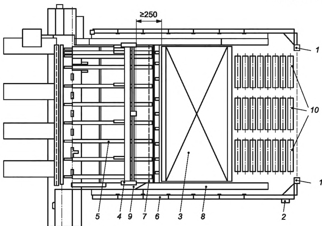
1 — AOPD 1; 2 — орган управления сбросом для AOPD 1; 3 — подъемная платформа; 4 — толкатель панели; 5 — опора для заготовки станка; 6 — боковые ограждения; 7 — AOPD 2; 8 — механический кулачок; 9 — переключатель положения; 10 — опциональные задние роликовые накопительные конвейеры
