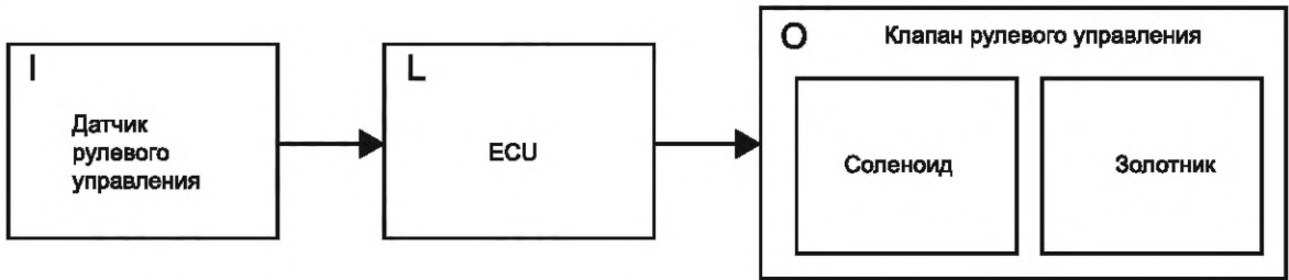
Рисунок А.2 — Логическая схема электрогидравлического рулевого управления категории В
