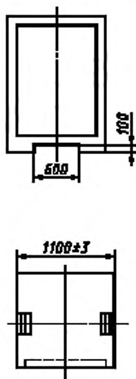
Контейнер типоразмера АУК-0,625
