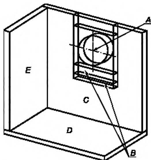
A — осевая линия соединительного элемента; B — вставки; C — задняя стенка; D — пол испытательного уголка; E — боковая стена
