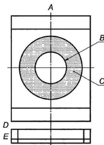
A — вид спереди; B — соединительная труба; C — изоляционный материал ( 150 \pm 5 ) мм вокруг соединительной трубы; D — аналогично конструкции на рисунке А.3; E — вид сверху
