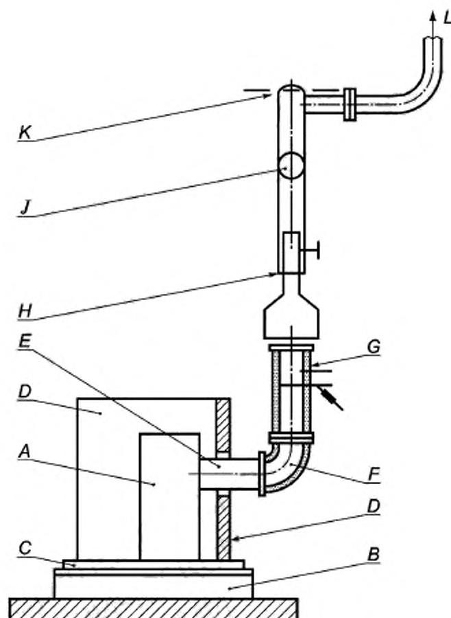
А — топка; G — измерительный участок, В — весовой помост, H — регулируемая часть трубы; C — днище; J — регулируемое сужающее устройство; D — боковая стенка; K — вентилятор; E — соединительный элемент; L — выпуск в атмосферу; F — переходное устройство
