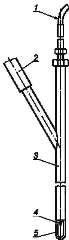
1 — подключение к измерительному прибору для измерения содержания \text{CO}_2 и температуры продуктов сгорания; 2 — подключение к откачивающему насосу; 3 — измерительный зонд; 4 — термолара, 5 — защита для наконечника термолары
