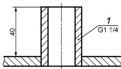
1 — газовая труба
