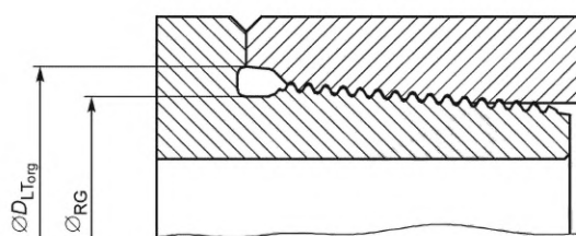
Рисунок 11 — Малый крутящий момент соединения
