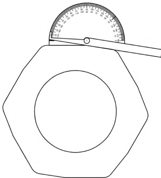
Рисунок 18 — Измерение угла износа ведущей или рабочей трубы
