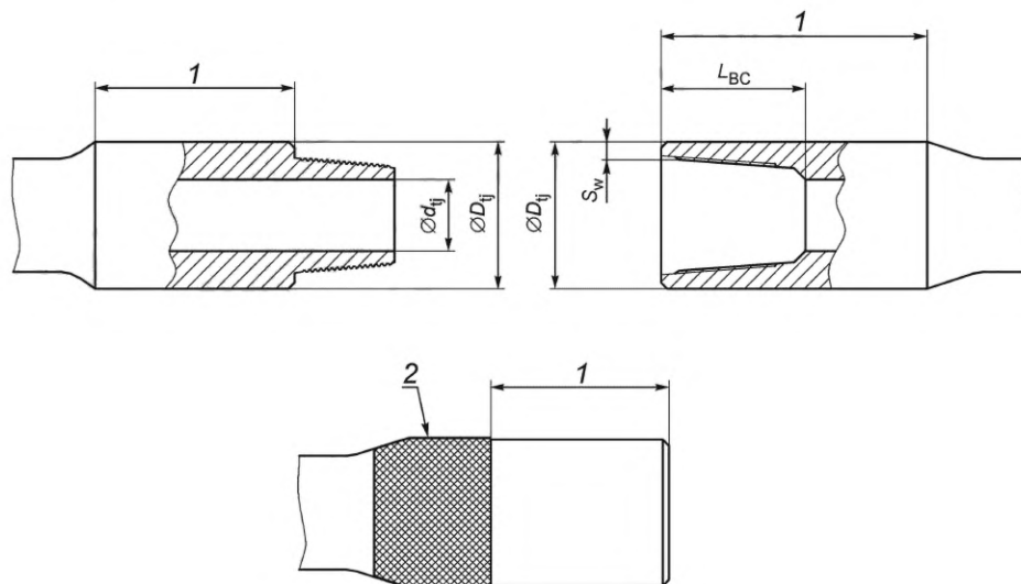
1 — место установки ключа; 2 — армирование/наплавка твердым сплавом
