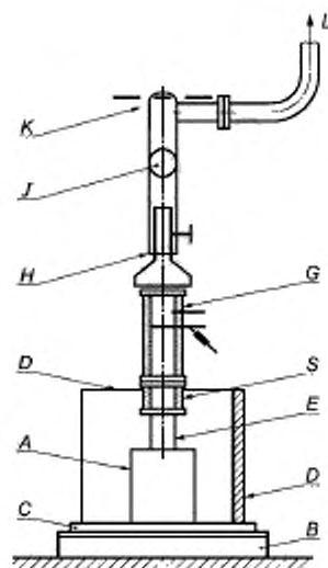
А — отопительный прибор; В — платформенные весы контроля выгорания топлива; С — пол испытательного угла; D — боковая стенка испытательного угла; E — дымоход; G — измерительный участок; H — регулируемая часть трубы; J — регулируемая дроссельная заслонка; K — вентилятор; L — выпуск в атмосферу; S — переходник для дымовых газов (прямой)
