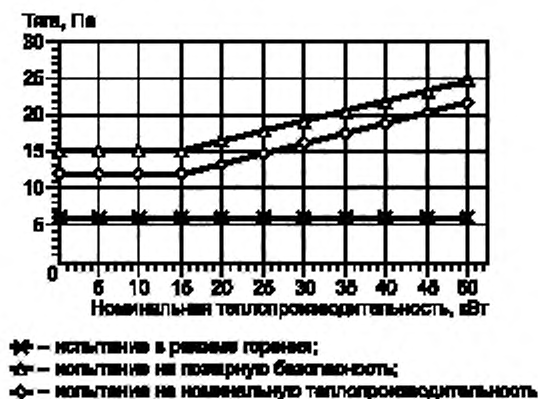
Рисунок 1 — Значения тяги в дымоходе
