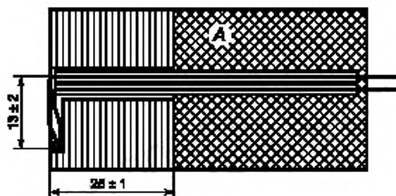
A — Стенка испытательного угла
