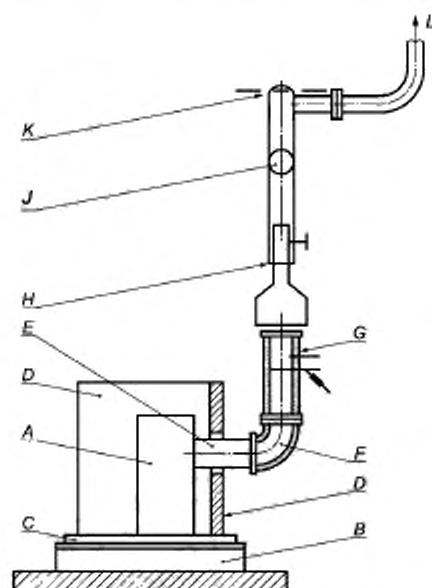
А — отопительный прибор; В — платформенные весы контроля выгорания топлива; С — пол испытательного угла; D — боковая стенка испытательного угла; E — дымоход; F — переходник для дымовых газов (колесо); G — измерительный участок; H — регулируемая часть трубы; J — регулируемая дроссельная заслонка; K — вентилятор; L — выпуск в атмосферу
