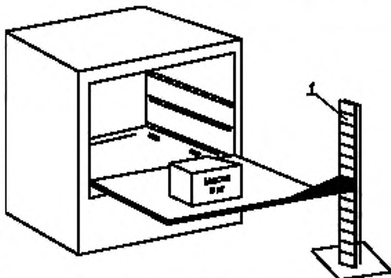
1 — датчик с измерительной линейкой
