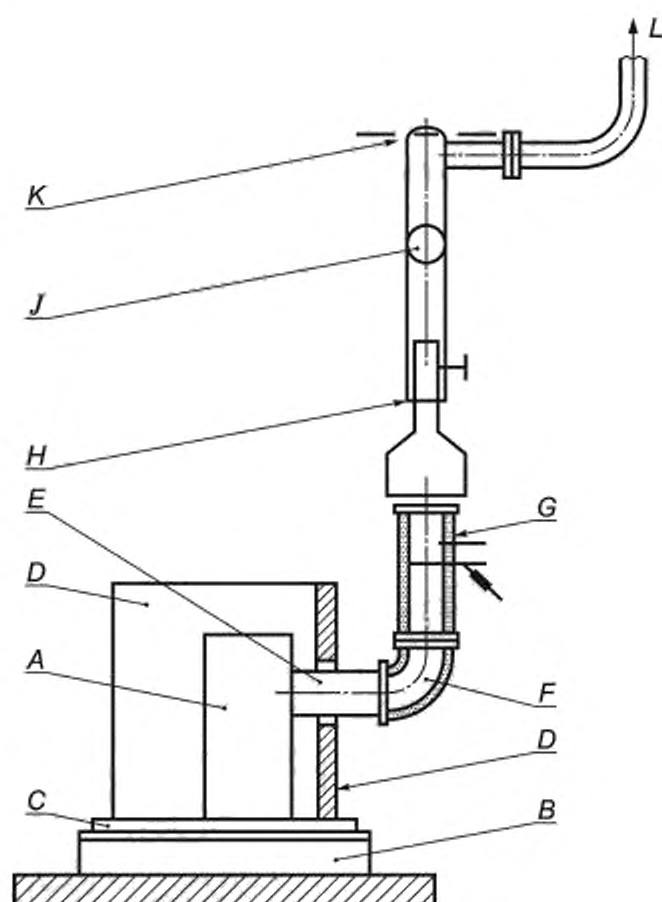
А — отопительный прибор; В — платформенные весы контроля выгорания топлива; С — пол испытательного угла; D — боковая стенка испытательного угла; E — дымоход; F — переходник для дымовых газов (колено); G — измерительный участок; H — регулируемая часть трубы; J — регулируемая дроссельная заслонка; K — вентилятор; L — выпуск в атмосферу
