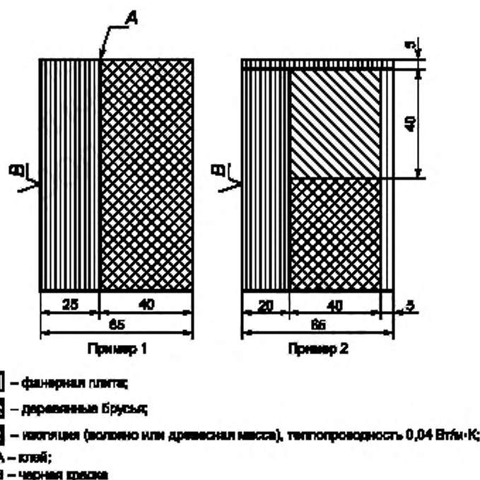
Рисунок А.5 — Разрез конструкции испытательного угла
