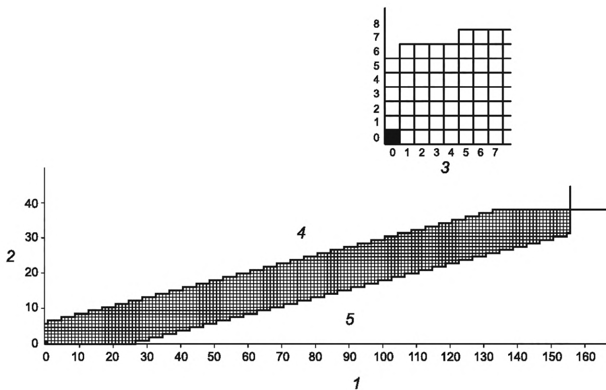
Рисунок В.2 — График испытания упаковки методом последовательных испытаний с участием детей (полный период испытаний)
