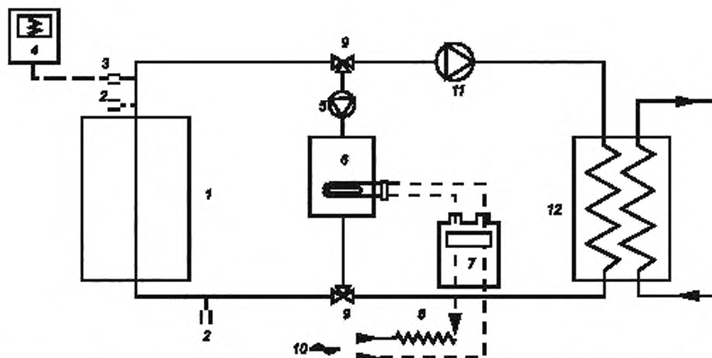
1 - испытуемый котел, 2 - датчик температуры, 3 - низкоинерционный термозлемент; 4 - записывающее устройство; 5 - насос (обеспечивает перепад температур между обоими термодатчиками в пределах 2 °С - 4 °С от максимальной испытательной температуры); 6 - электрический водонагреватель; 7 - электросчетчик; 8 - регулятор напряжения, 9 - клапан на 1/4 поворота, 10 - электропитание, 11 - вспомогательный насос (при необходимости); 12 - теплообменник
