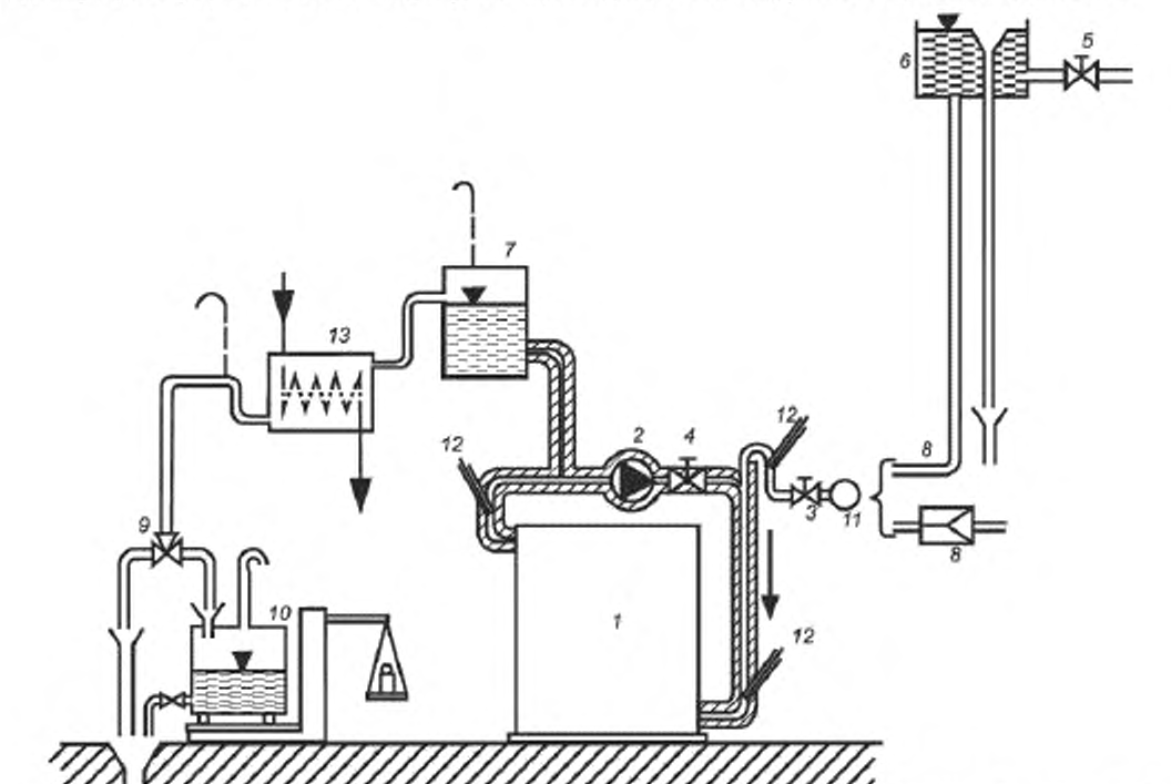
1 – испытуемый котел, 2 – циркуляционный насос, 3 – управляющий клапан I, 4 – управляющий клапан II, 5 – управляющий клапан III, 6 – бак постоянного напора, 7 – компенсационный бак, 8 – подсос к распределительной трубе постоянного давления, 9 – трехходовой кран, 10 – сосуд для взвешивания, 11 – счетчик для воды, 12 – термометры, 13 – охладитель Рисунок 1 — Испытательный стенд с прямой циркуляцией
