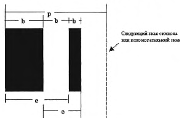
Рисунок F.1 — Размеры для определения допусков
