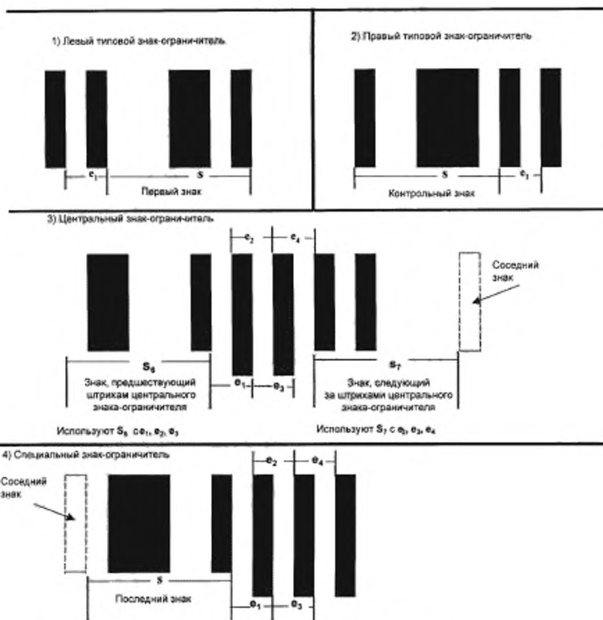
Рисунок 8 — Размеры вспомогательных знаков
