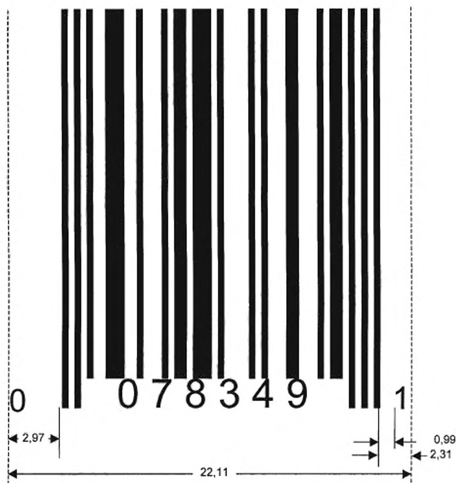
Рисунок E.5 — Символ UPC-E
