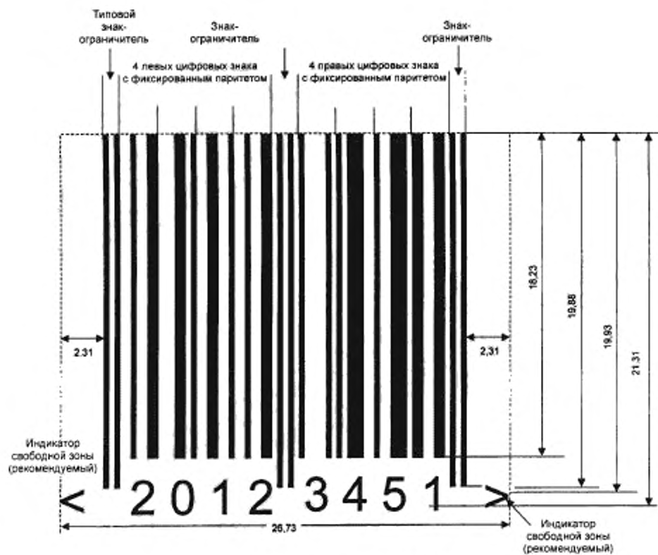
Рисунок E.4 — Символ EAN-8
