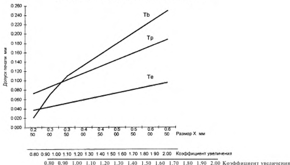
Рисунок F.2 — Допуски, рассчитанные для различных значений X
