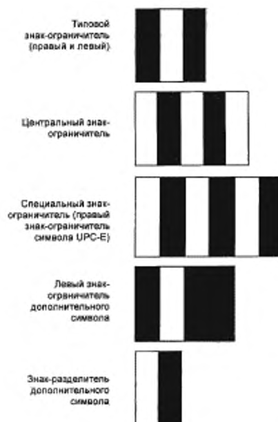
Рисунок D.2 — Представление вспомогательных знаков
