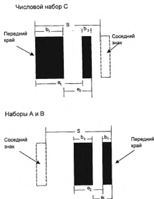
Рисунок 7 — Размеры декодирования знаков символов
