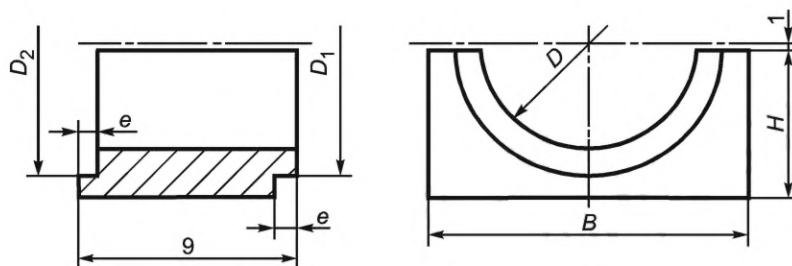
Рисунок 3 — Изделия №№ 1-а, 1-б, 2-а, 2-б, 3-а, 3-б, 4-а, 4-б, 5-а, 5-б, 6-а, 6-б, 7-а, 7-б, 8-а, 8-б, 9-а, 9-б, 10-а, 10-б (Удлинительное кольцо)
