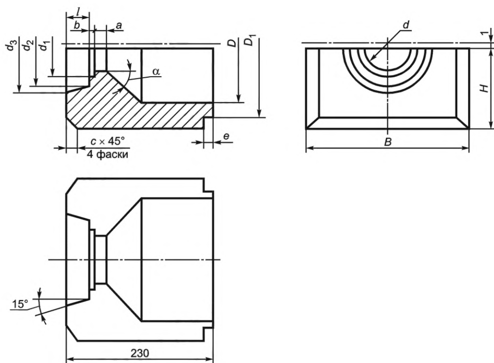
Рисунок 2 — Изделия №№ 1-2, 2-2, 3-2, 4-2, 5-2, 6-2, 7-2, 8-2, 9-2, 10-2 (Камера. Тип 2)
