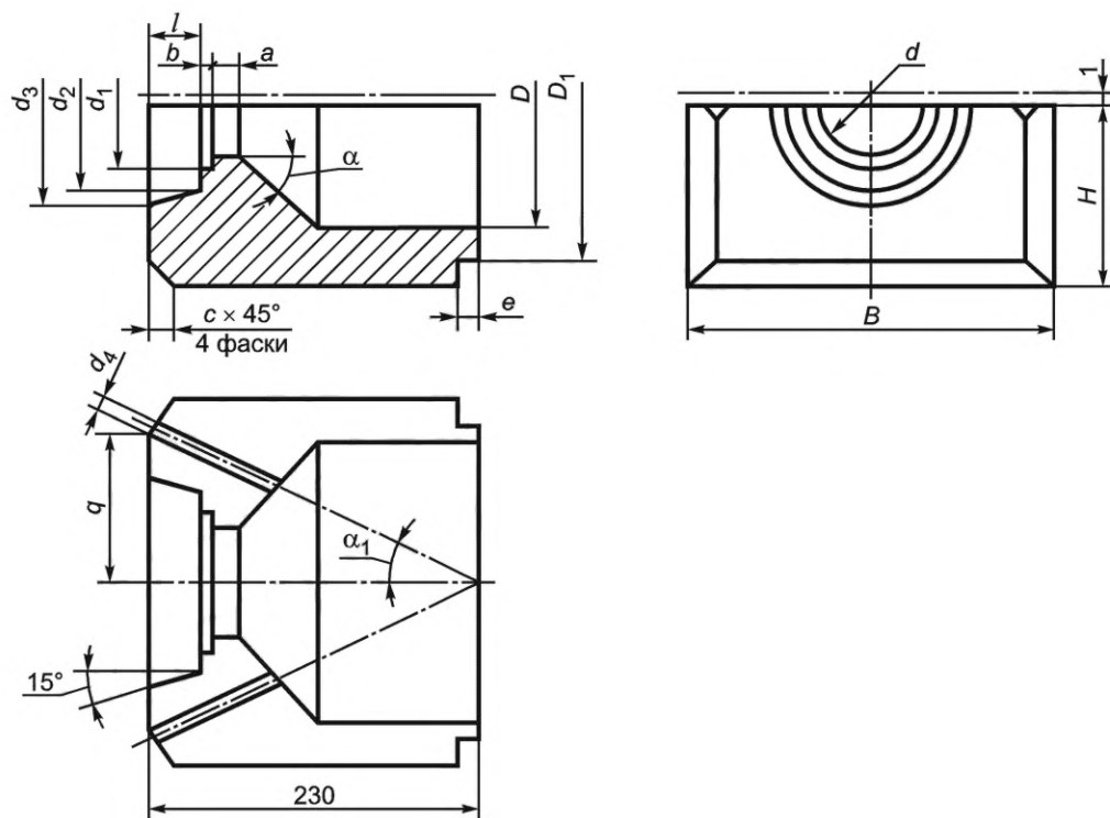
Рисунок 1 — Изделия №№ 1-1, 2-1, 3-1, 4-1, 5-1, 6-1, 7-1, 8-1, 9-1, 10-1 (Камера. Тип 1)
