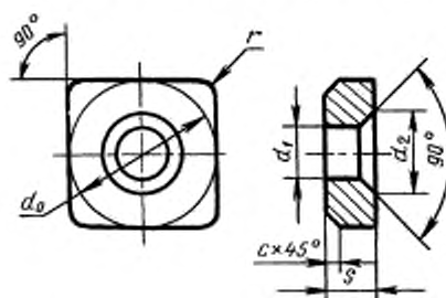
Размеры, мм
