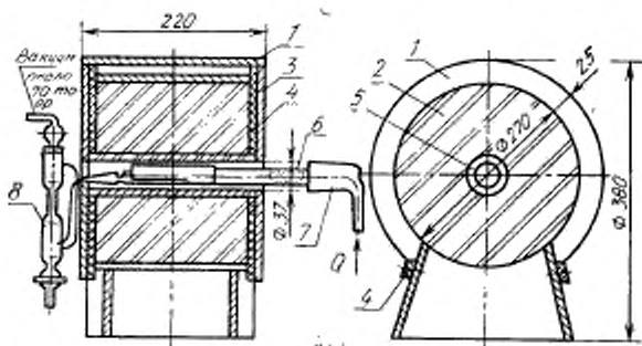
1 — алюминиевая металлическая обшивка (открыта сбоку); 2 — изольдур; 3 — алюминиевый боковой лист; 4 — асбест; 5 — керамическая трубка; 6 — кварцевая трубка для сжигания; 7 — форштос; 8 — абсорбционный сборник
