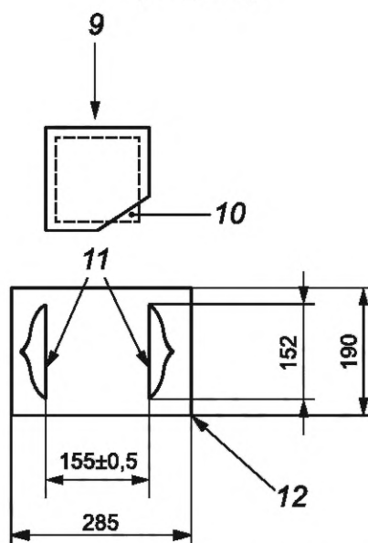
б) Элементы держателя испытываемой пробы с типовыми размерами
