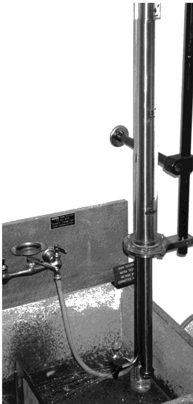
Рисунок 1 — Устройство для испытания методом дождевания, полная сборка
