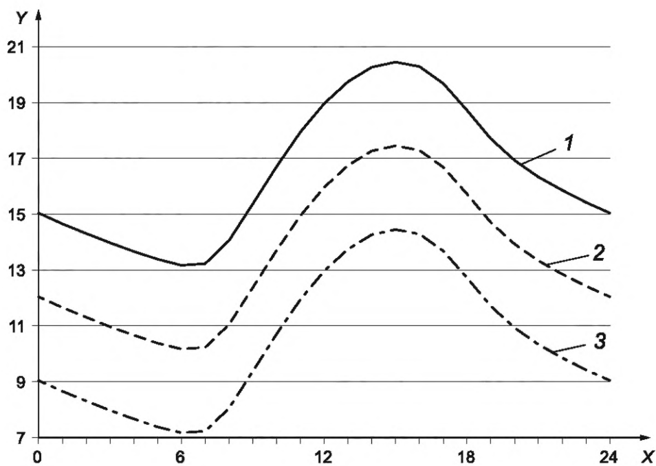
Рисунок А.2 — Пример температурного режима внешней среды в зимний сезон
