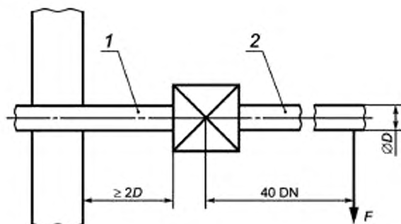
1 — труба 1; 2 — труба 2; D — внешний диаметр; F — сила
