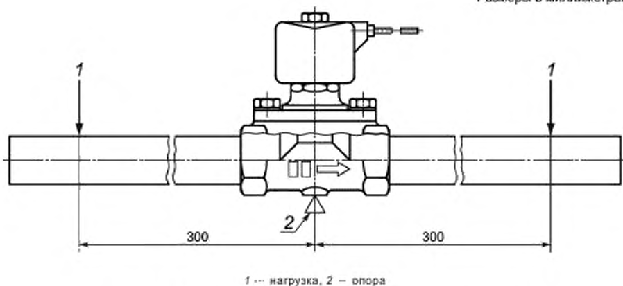
Рисунок G.1 — Устройство для испытания изгибающего момента
