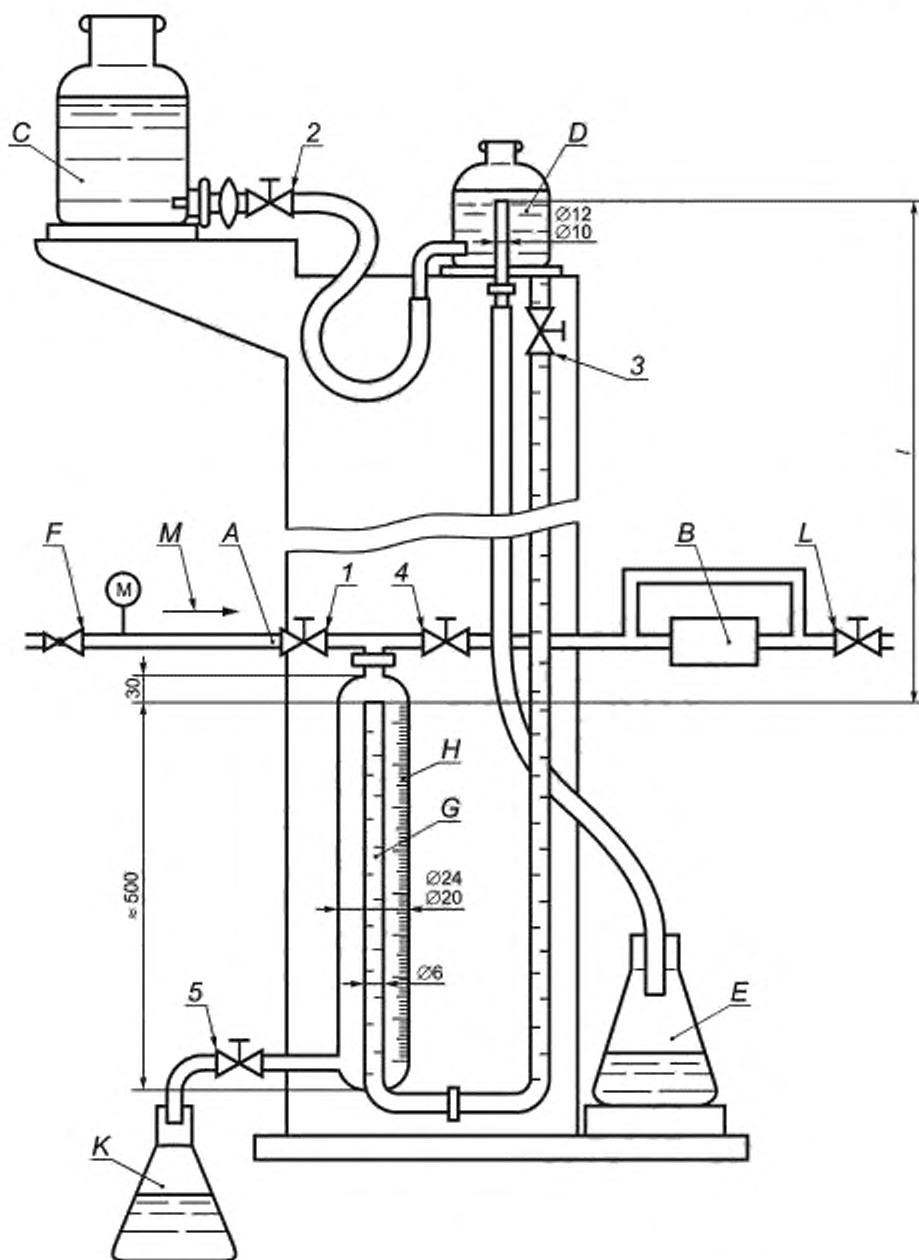
A — входное отверстие; B — образец испытания; C — емкость для воды; D — колба с постоянным уровнем; E — расширительный бак; F — регулятор; G — труба; H — измерительная бюретка; K — водоотвод; L — выпускной кран; M — сжатый поток воздуха; от 1 до 5 — краны ручного управления
