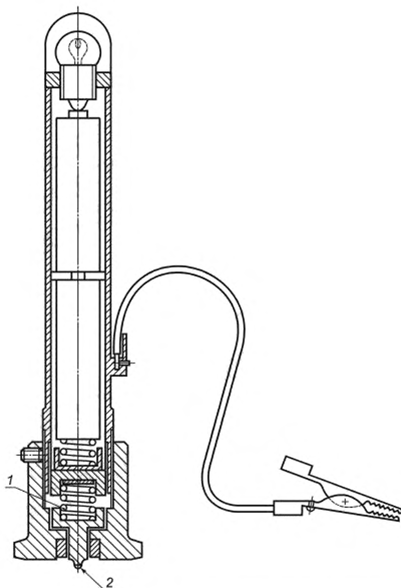
1 — нагрузка за счет сжатия пружины (10 Н); 2 — точка царапины (стальной шар, диаметром 1 мм)
