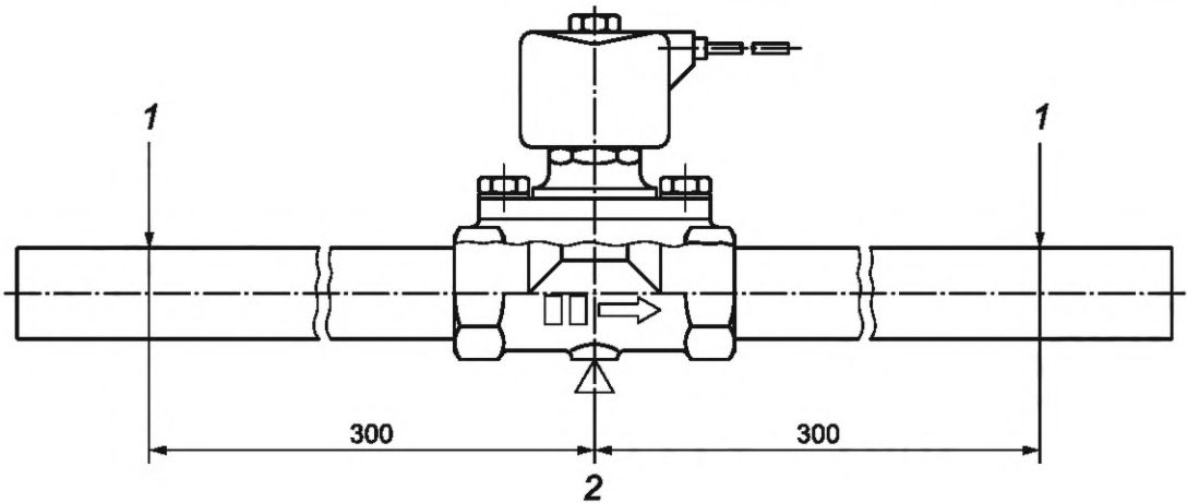
1 — нагрузка; 2 — ось
