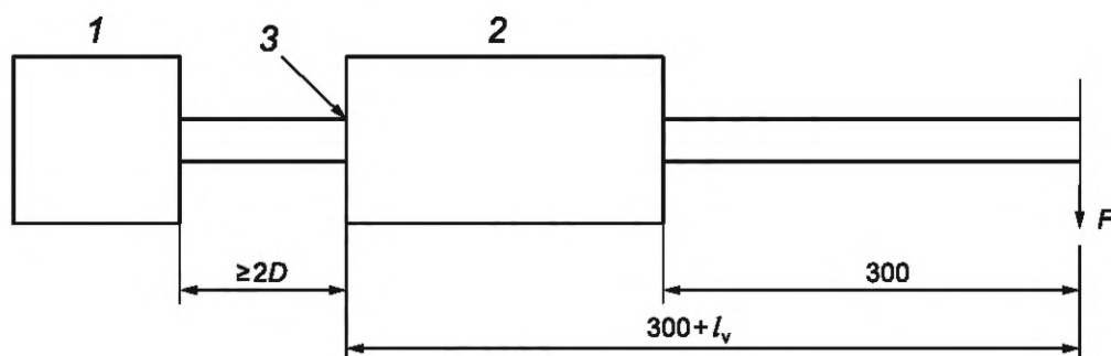
Рисунок 4 — Устройство для испытания на изгиб
