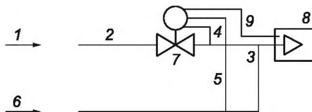
Рисунок I.5 — Регулятор расхода (поступное регулирование расхода/подогретый воздух)
