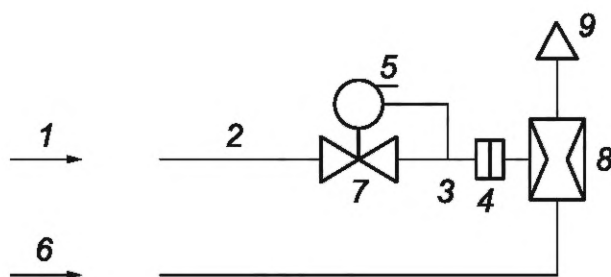
Рисунок I.3 — Контроль соотношения воздух/газ (регулятор плавного действия)
