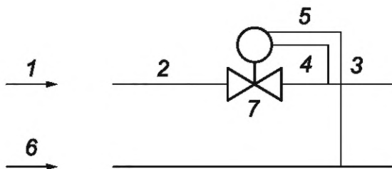
Рисунок I.2 — Редуктор давления с дополнительной энергией (управление в режиме постоянного давления)
