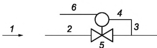
Рисунок I.1 — Редуктор давления (управление в режиме постоянного давления)
