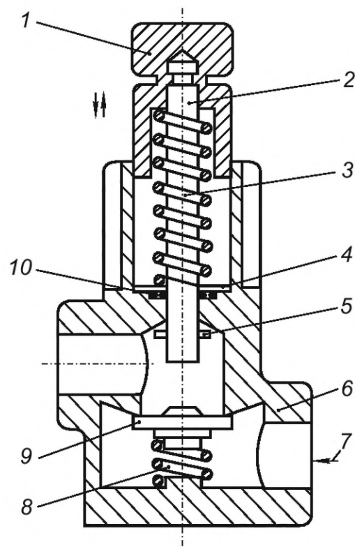
1 — рабочий шпindel; 2 — шток клапана; 3 — пружина для рабочего шпинделя; 4 — шайба; 5 — остановка шпинделя; 6 — корпус клапана; 7 — вход; 8 — дисковая пружина; 9 — диск клапана; 10 — уплотнительное кольцо
