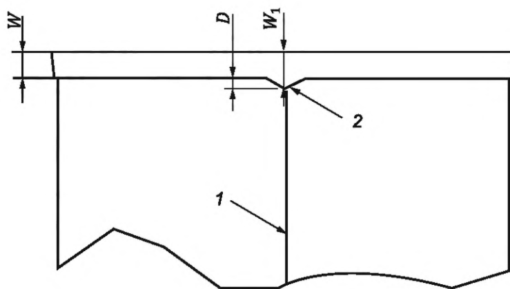
1 — сварной шов; 2 — наклон
