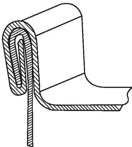
Рисунок 8 — Заостренный шов
