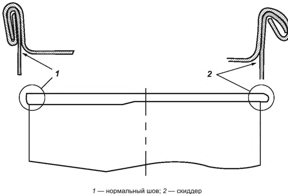
Рисунок 2 — Пустое место; вращатель; скиддер; скользящий закаточный шов
