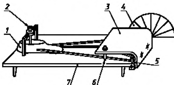
1 — ласта; 2 — прижимной винт; 3 — изгибающая пластина; 4 — транспорт; 5 — ось; 6 — шпилька; 7 — основание
