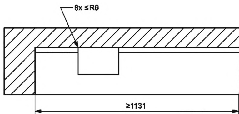
Рисунок 3 — Интерфейс сменного оборудования — Разрез А—А (рисунок 2)
