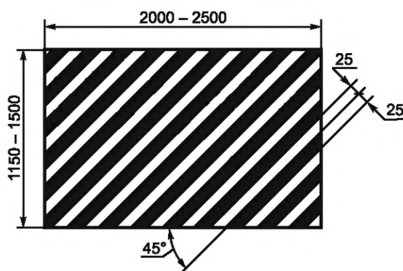
Рисунок 1 — Экран «зебра»
