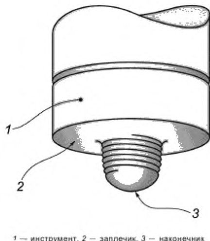
Рисунок 9 — Инструмент для сварки трением с перемешиванием
