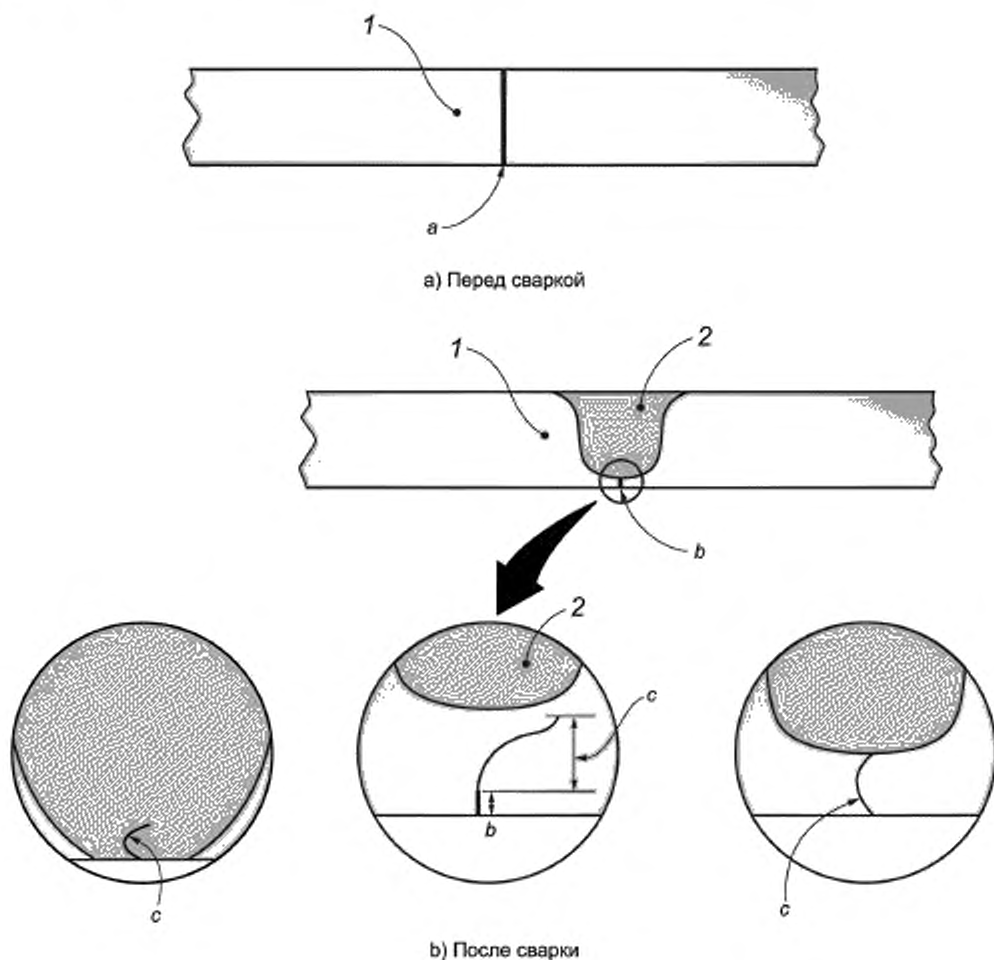
1 — деталь, 2 — сварной шов; а — стык (сопрягаемые поверхности), б — непровар — пластическая деформация отсутствует; в — непровар — сильная пластическая деформация (слипание)
