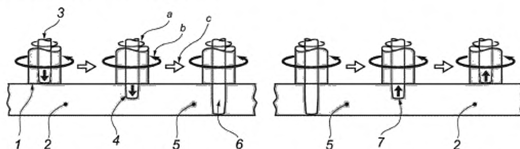
1 — заплечик; 2 — свариваемая деталь; 3 — наконечник; 4 — наконечник, движущийся вниз; 5 — сваренная деталь; 6 — наконечник в требуемом положении для сварки; 7 — наконечник, движущийся вверх; a — направление вращения наконечника; b — направление вращения заплечика; c — направление сварки
