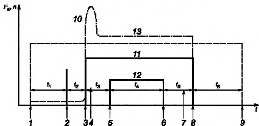
F_a — осевое усилие; n — частота вращения инструмента; t — время; t_1, t_2, t_3, t_4, t_5, t_6 — время действия; 1 — начало вращения; 2 — движение инструмента к детали; 3 — касание инструмента детали; 4 — время выдержки в начале сварного шва; 5 — начало линейного движения; 6 — остановка линейного движения; 7 — время выдержки в конце сварного шва; 8 — движение инструмента от детали; 9 — остановка вращения; 10 — возрастание осевого усилия; 11 — сварка деталей; 12 — линейное движение инструмента; 13 — постоянное осевое усилие
