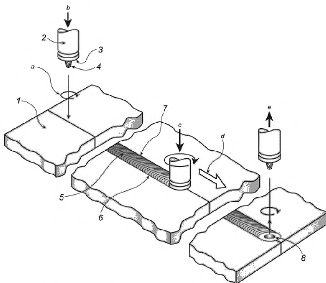
1 — деталь, 2 — инструмент; 3 — заплечик, 4 — наконечник; 5 — лицевая сторона шва; 6 — сторона отставания шва; 7 — сторона набегания шва, 8 — выходное отверстие, а — направление вращения инструмента; b — движение инструмента вниз, c — осевое усилие; d — направление сварки; e — движение инструмента вверх
