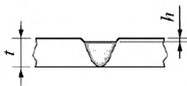
h — глубина неполного заполнения; t — толщина
